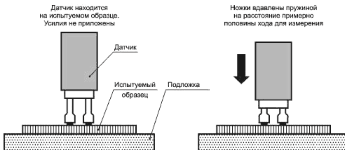
Рисунок 4 — Сжатие пружин при измерении
