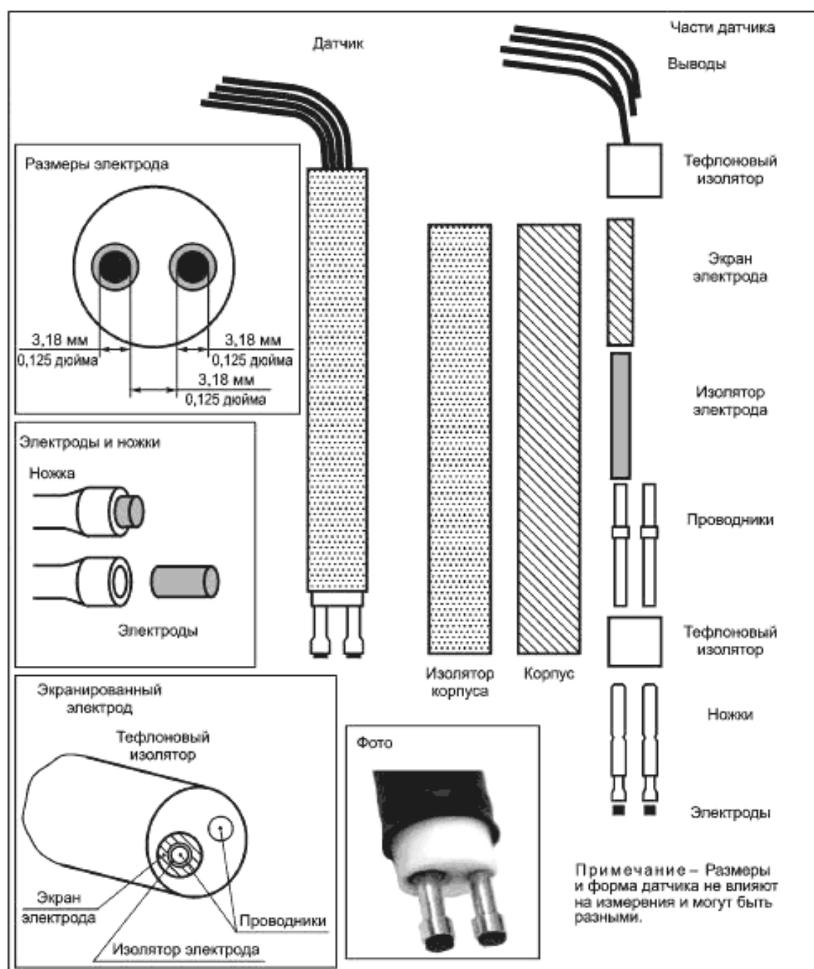
Рисунок 1 — Конфигурация двухконтактного датчика
