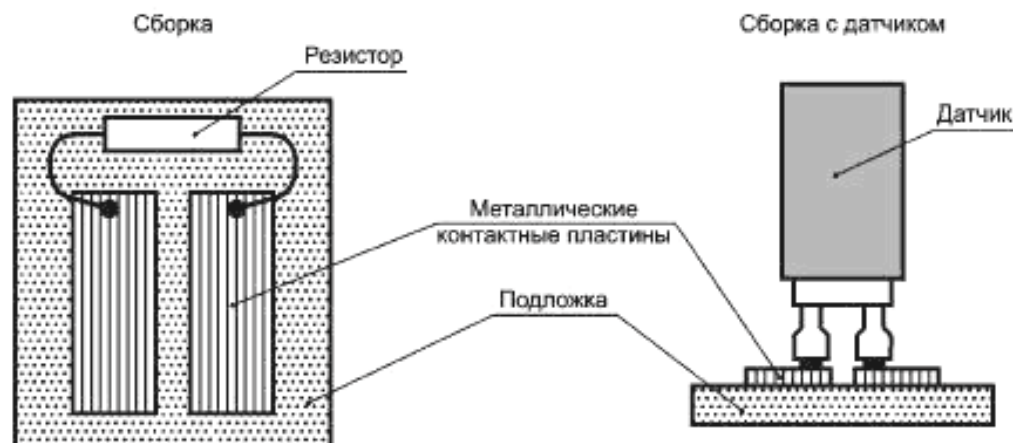
Рисунок 3 — Сборка для проверки сопротивления
