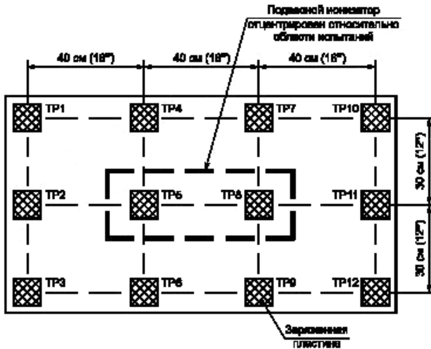
Рисунок 13. Области испытаний подвешенного ионизатора (вид сверху)
