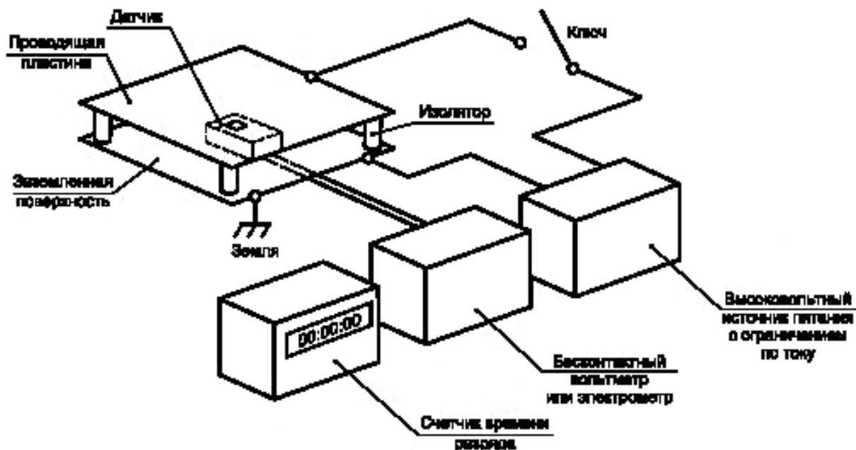
Рисунок 1 – Схема подключения измерительной пластины
