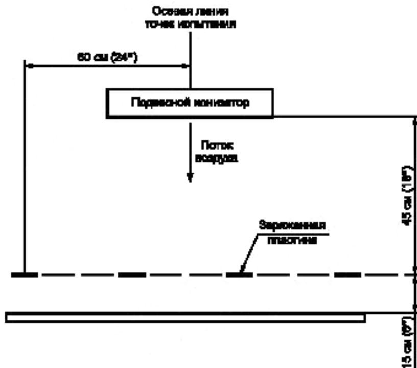
Рисунок 14. Области испытаний подвешенного ионизатора (вид сбоку)
