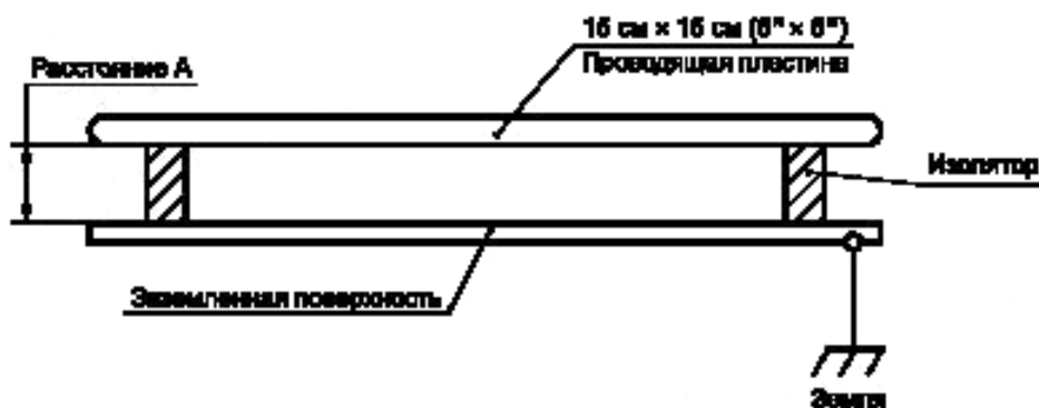
Рисунок 1 – Схема подключения измерительной пластины
