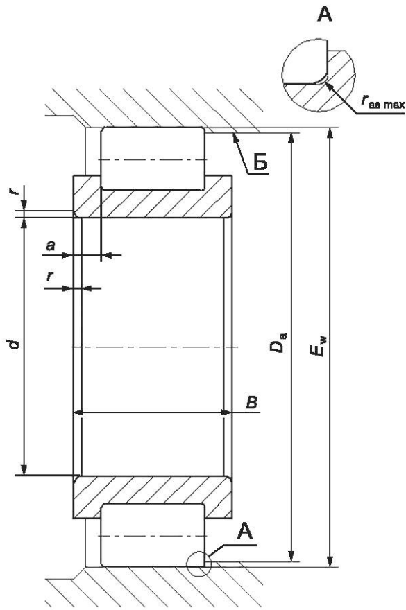
Рисунок 2 — Конструктивное исполнение 50
