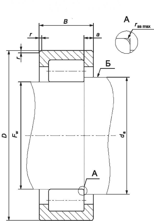
Рисунок 1 — Конструктивное исполнение 29
