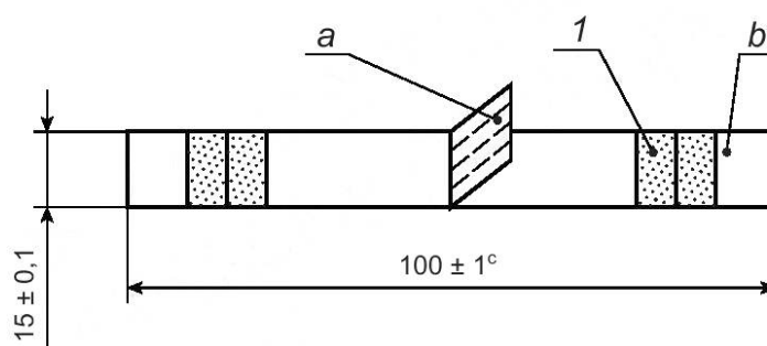
Рисунок 2 — Схема отбора образцов для испытания прочности сварных швов
