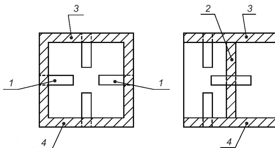
Рисунок 2 — Схема отбора образцов для испытания прочности сварных швов
