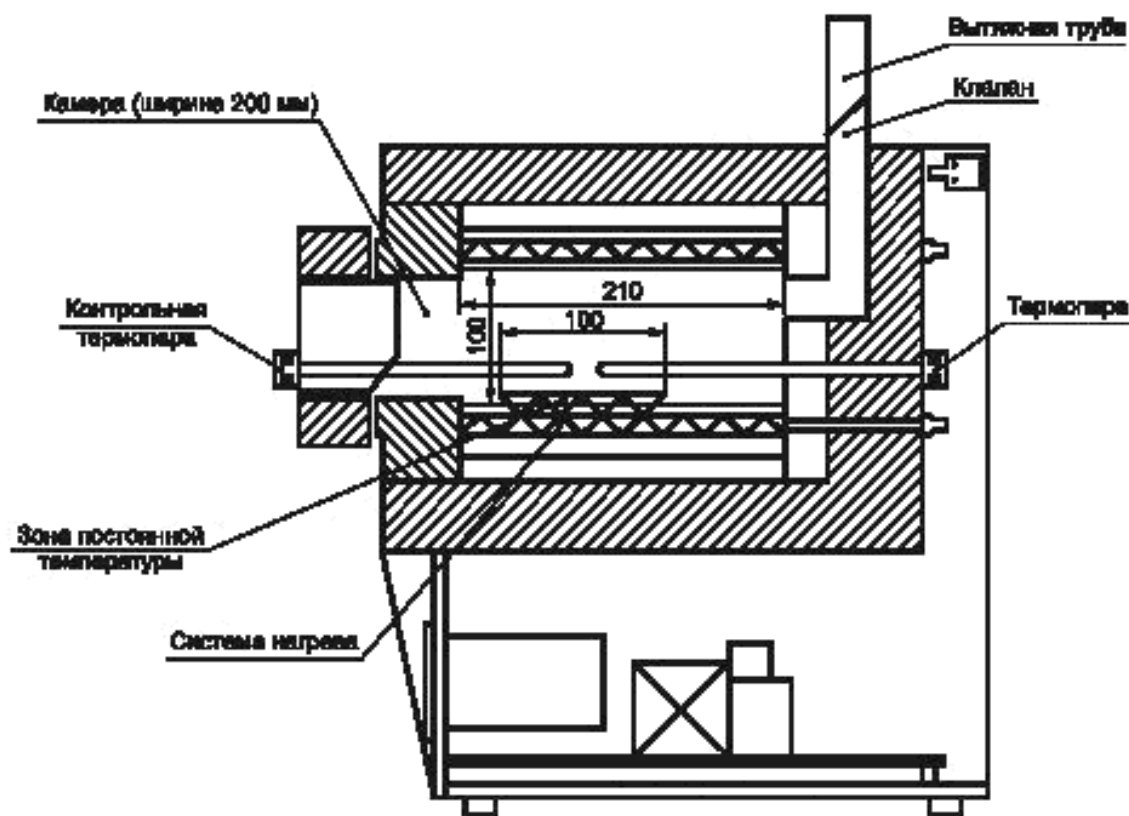
Рисунок 1 — Муфельная печь с электрообогревом (размеры даны в миллиметрах)
