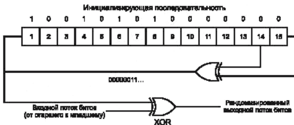
Рисунок 3 — Схема рандомизации данных
