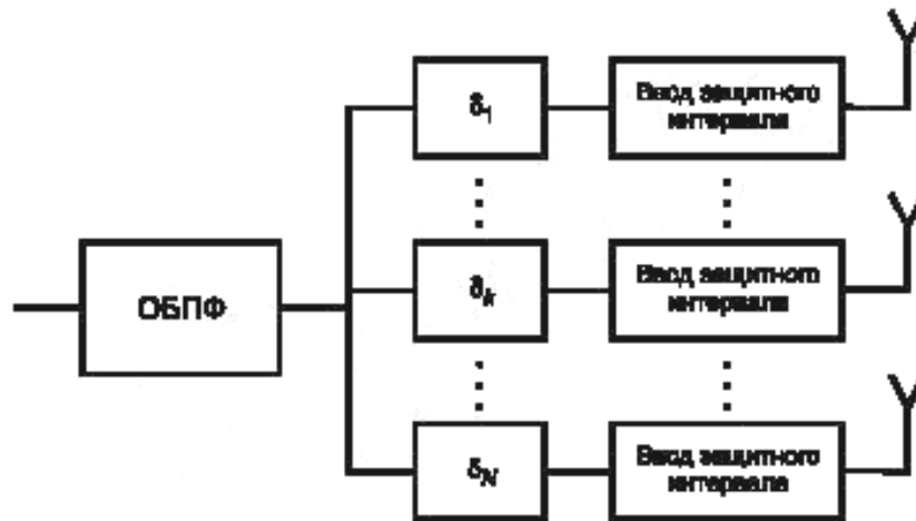
Рисунок Г.1 — Схема разнесенной передачи
