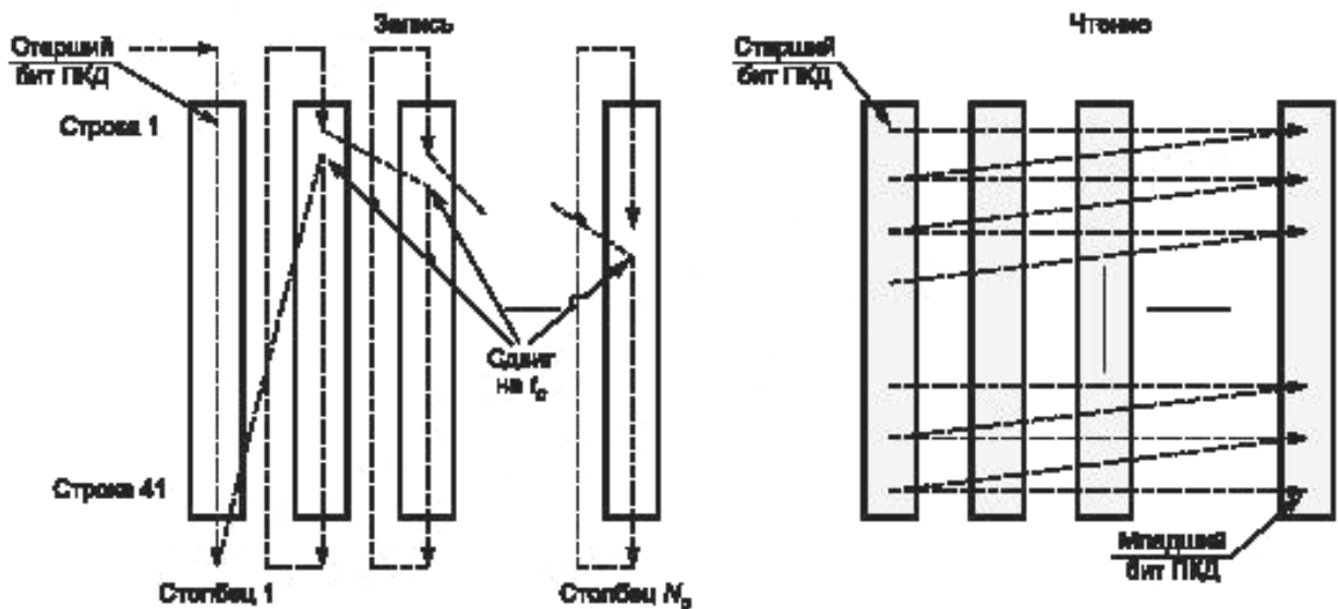
Рисунок 4 — Процедура битового перемежения
