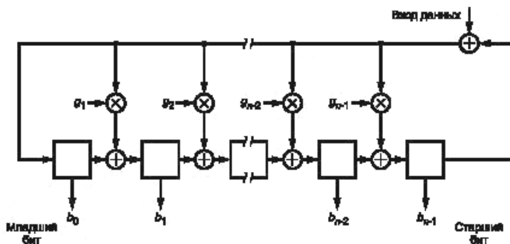
Рисунок Д.1 — Блок-схема вычисления CRC-кода
