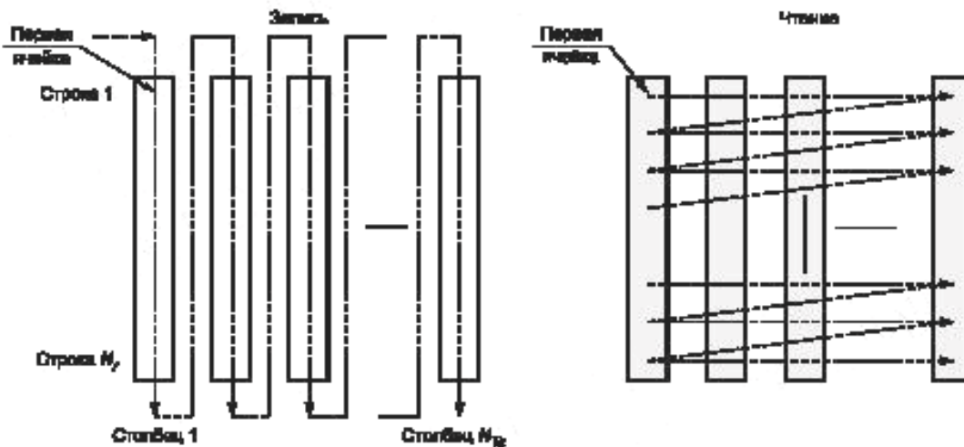
Рисунок 7 — Схема временного перемежителя
