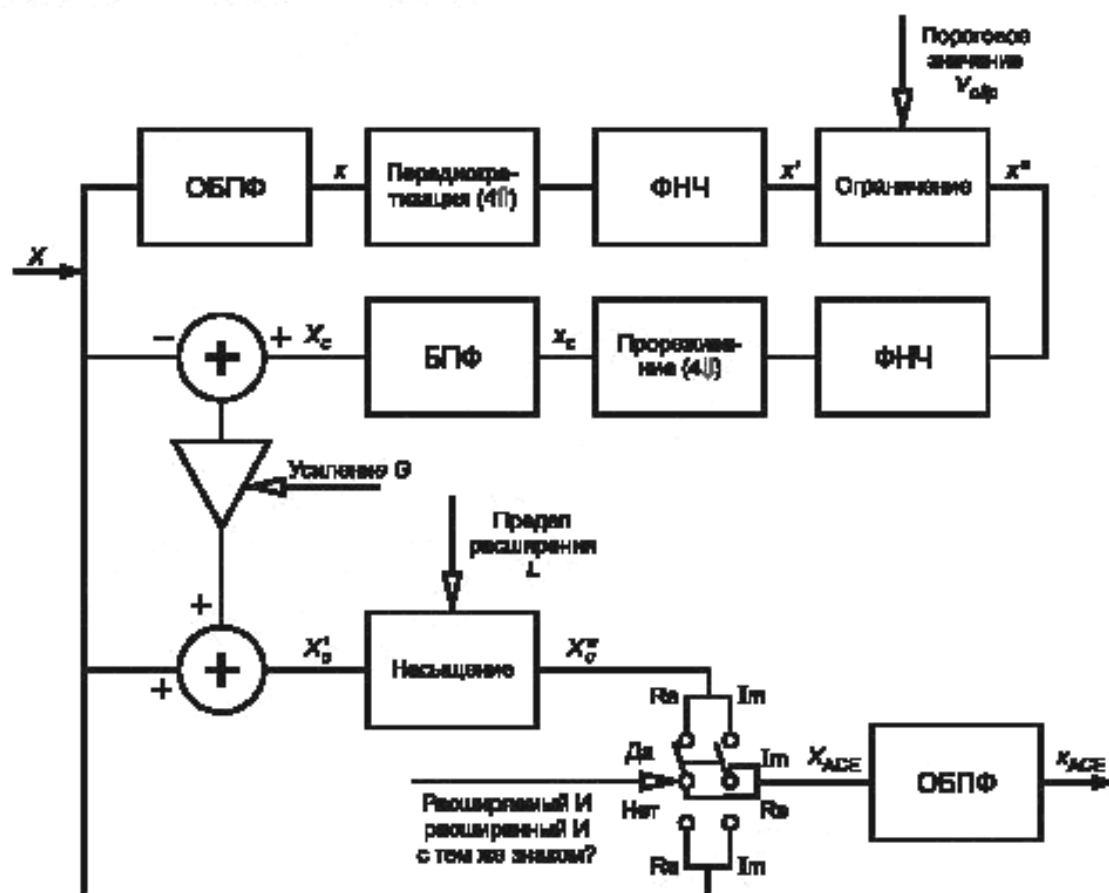
Рисунок В.1 — Схема алгоритма АСЕ
