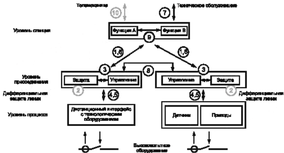
Рисунок ДА.1 — Модель интерфейсов системы автоматизации подстанции
