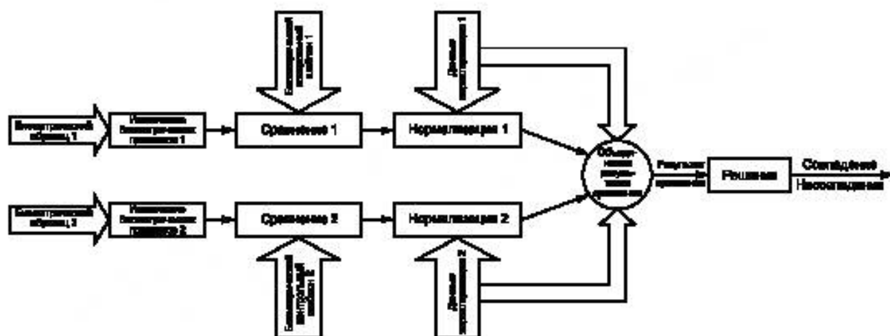
Рисунок 5 — Структура объединения на уровне результатов сравнения
