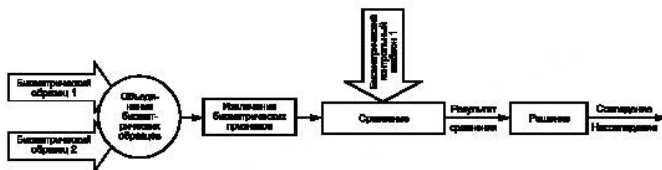
d) Объединение на уровне биометрических образцов
