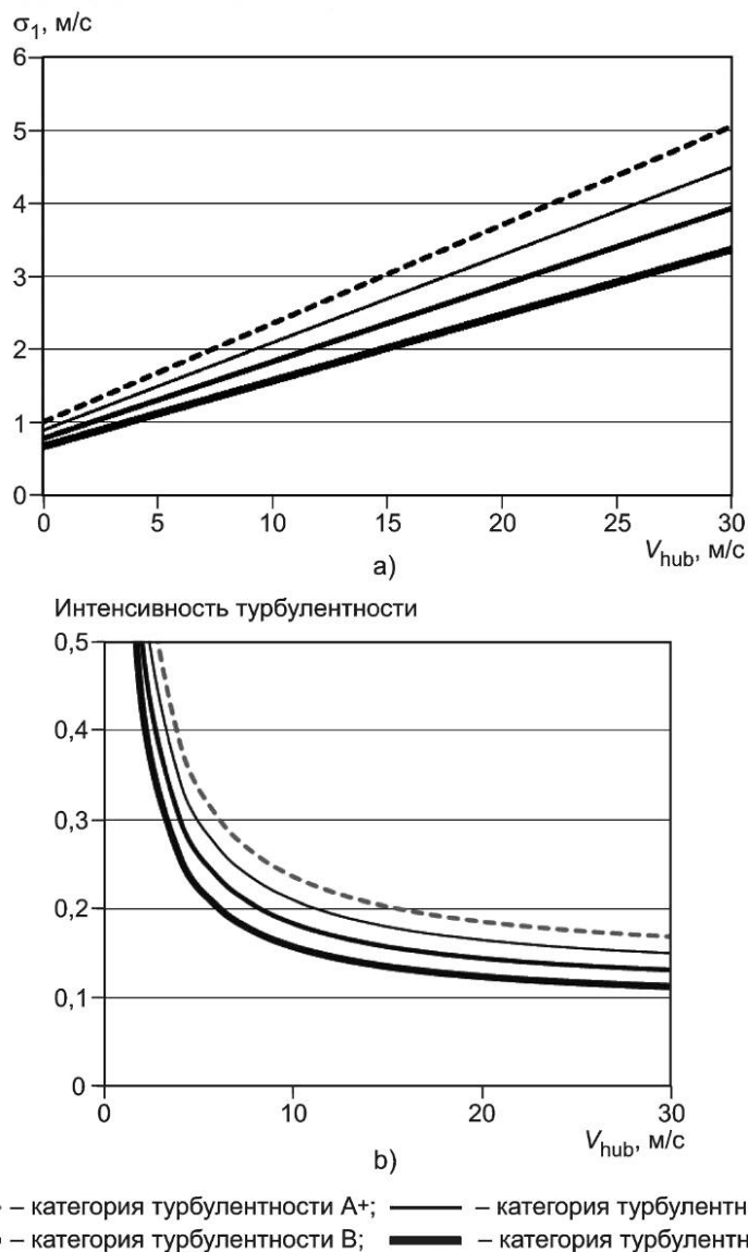
Рисунок 1 — Среднеквадратичное отклонение турбулентности (a) и интенсивность турбулентности (b) для модели нормальной турбулентности
