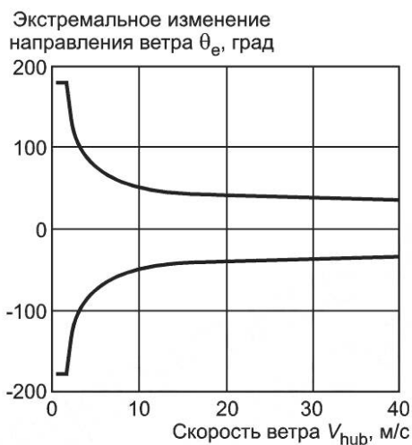
Рисунок 3 — Пример экстремальной величины изменения направления
