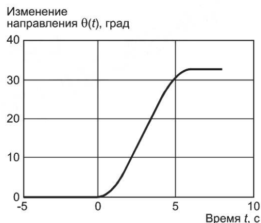
Рисунок 4 — Пример переходного процесса изменения направления
