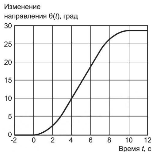
Рисунок 7 — Пример переходного процесса изменения направления
