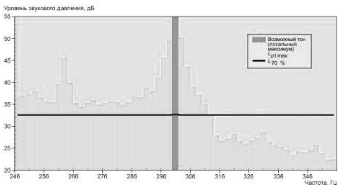
Рисунок 8 — Уровень L_{70\%} для одной критической полосы частот
