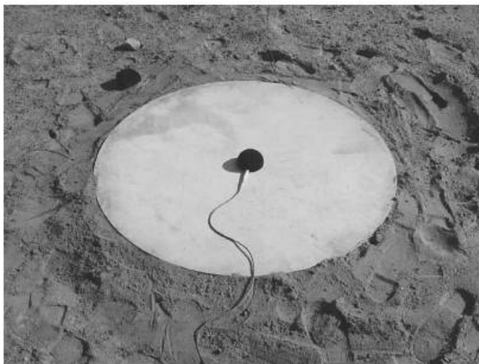
Рисунок 2 — Микрофон, установленный на измерительной панели
