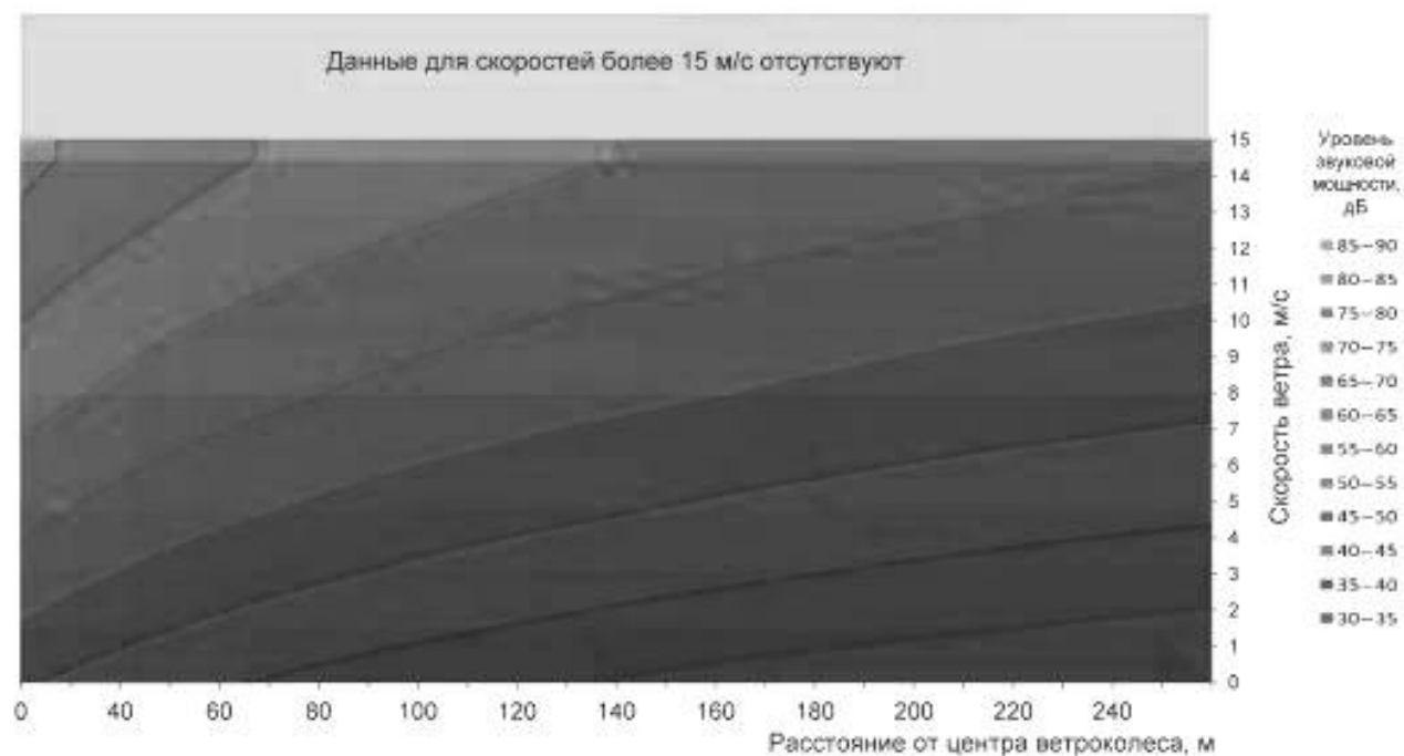
Рисунок Е.2 — Пример карты изолиний уровней звуковой мощности малой ветроустановки
