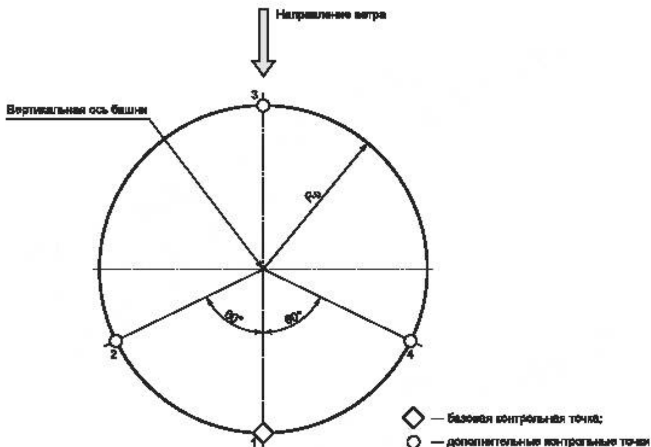
Рисунок 3 — Стандартные контрольные точки для размещения микрофона (вид сверху)
