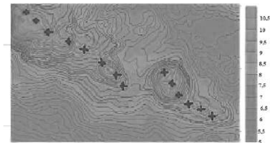
Рисунок В.5 – Диаграмма расчета распределения скорости ветра, [м/с] на территории ВЭС
