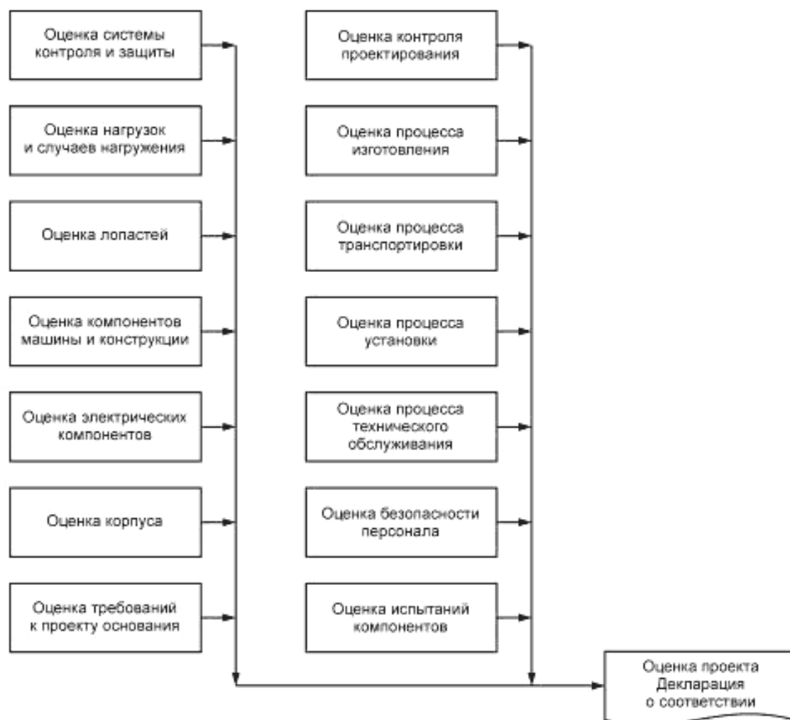
Рисунок 4 — Блок-схема процедуры оценки конструкции ВЭУ
