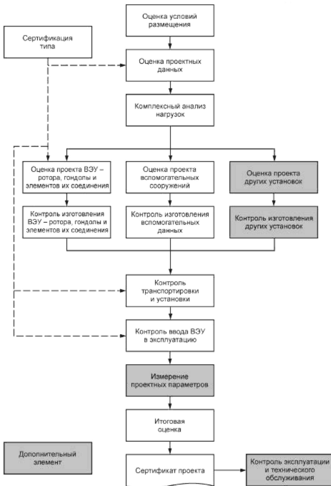
Рисунок 2 — Блок-схема процедуры сертификации проекта
