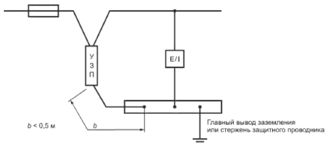
Рисунок F.1 — Двухточечная схема установки
