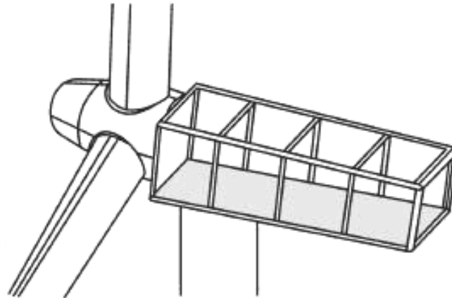
Рисунок E.2 — Сетка с большим размером ячеек для гондолы с кожухом из стеклопластика
