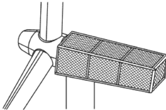
Рисунок E.3 — Сетка с маленьким размером ячеек для гондолы с кожухом из стеклопластика
