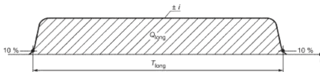
Рисунок А.4 — Определение параметров длинного удара молнии (обычно 2 \text{ мс} < T_{long} < 1 \text{ с} )
