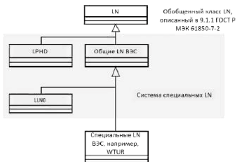
Рисунок 2 – Связь между логическими узлами
