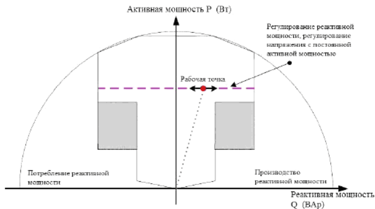
Рисунок В.9 – Схематическое изображение функции управления напряжением, используя регулирование реактивной мощности
