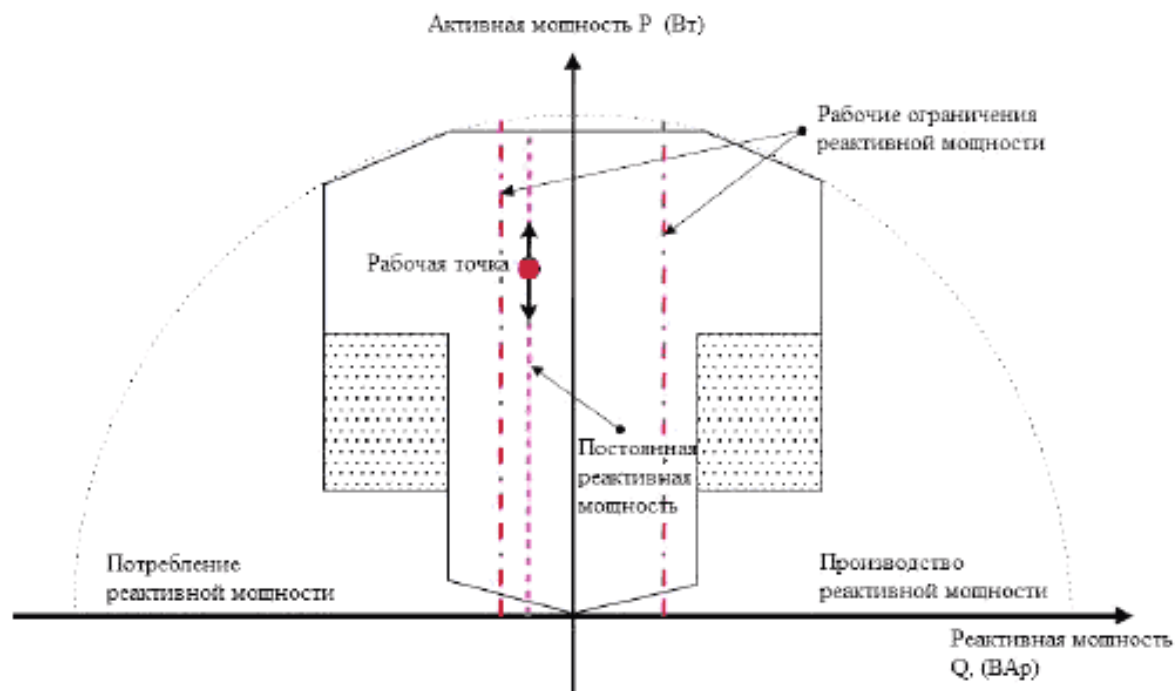
Рисунок В.7 – Схематическое изображение функции управления реактивной мощностью
