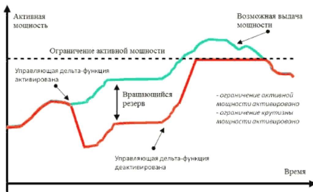
Рисунок В.4 – Схематическое изображение управляющей дельта-функции мощности
