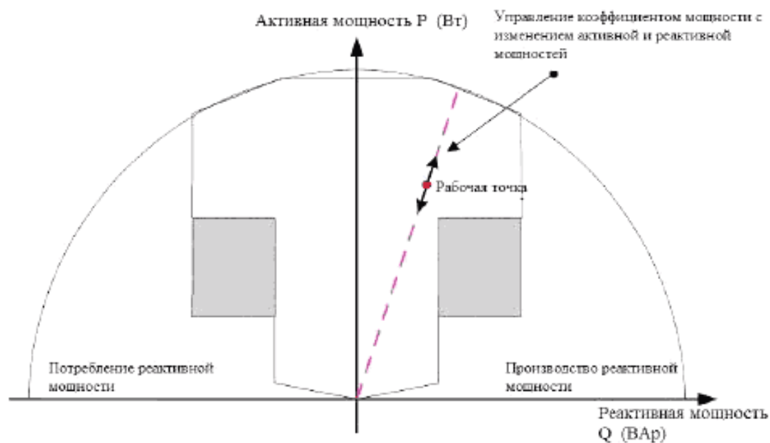
Рисунок В.8 – Схематическое изображение функции управления коэффициентом мощности
