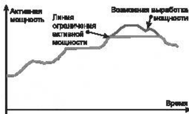
Рисунок В.2 – Схематическое изображение функции управления ограничением активной мощности
