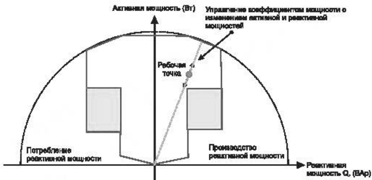
Рисунок В.8 – Схематическое изображение функции управления коэффициентом мощности
