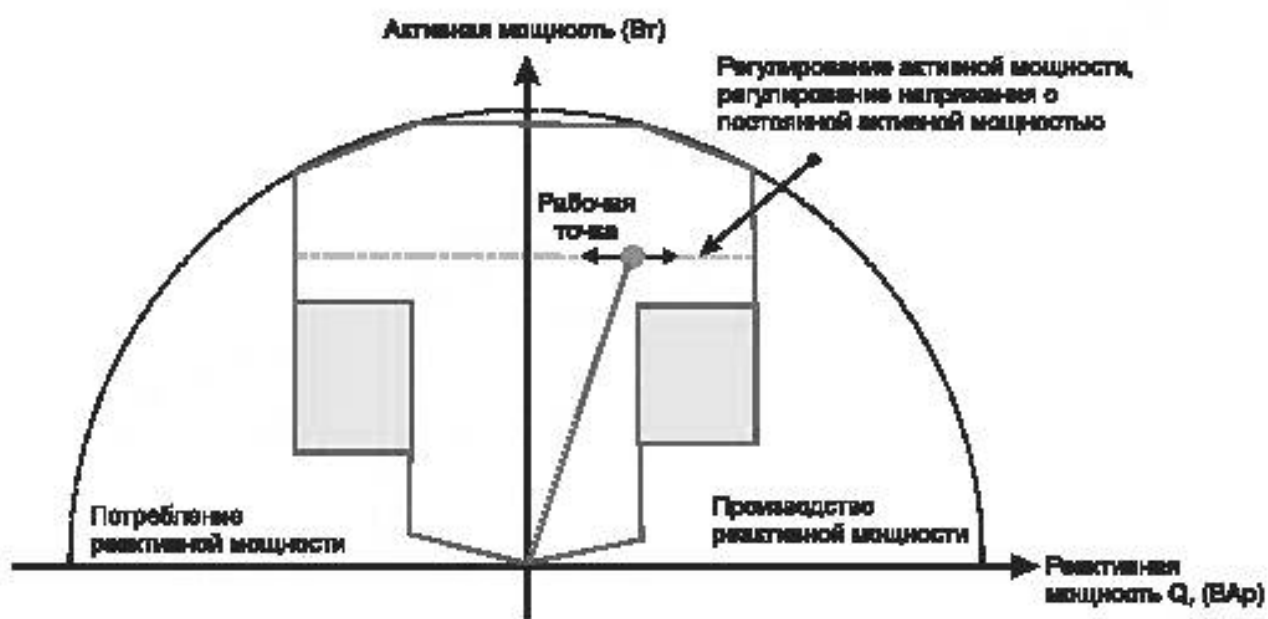
Рисунок В.9 – Схематическое изображение функции управления напряжением, используя регулирование реактивной мощности
