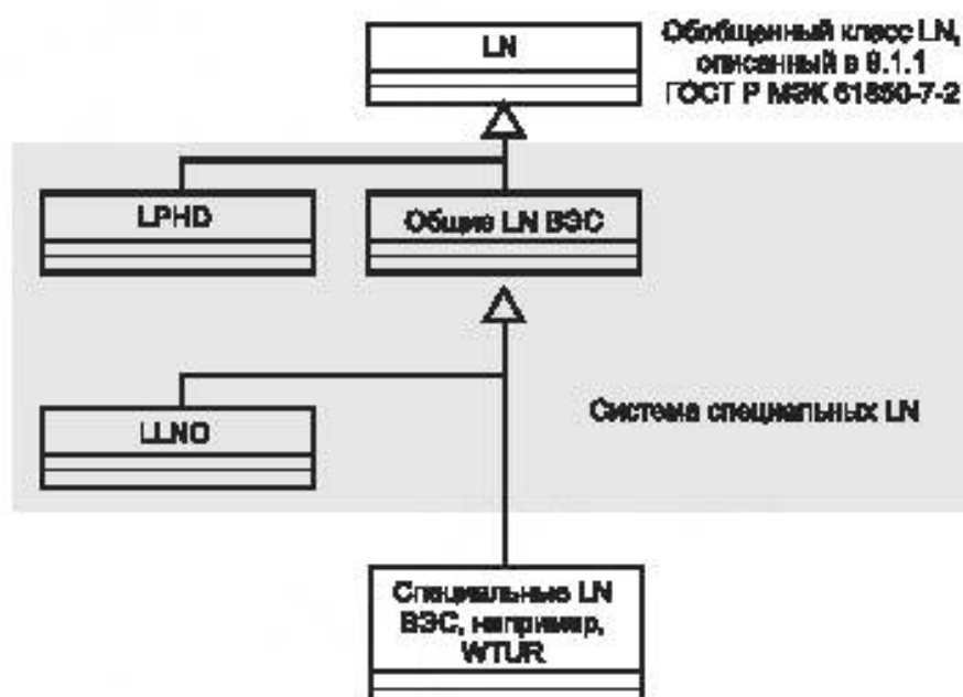
Рисунок 2 – Связь между логическими узлами
