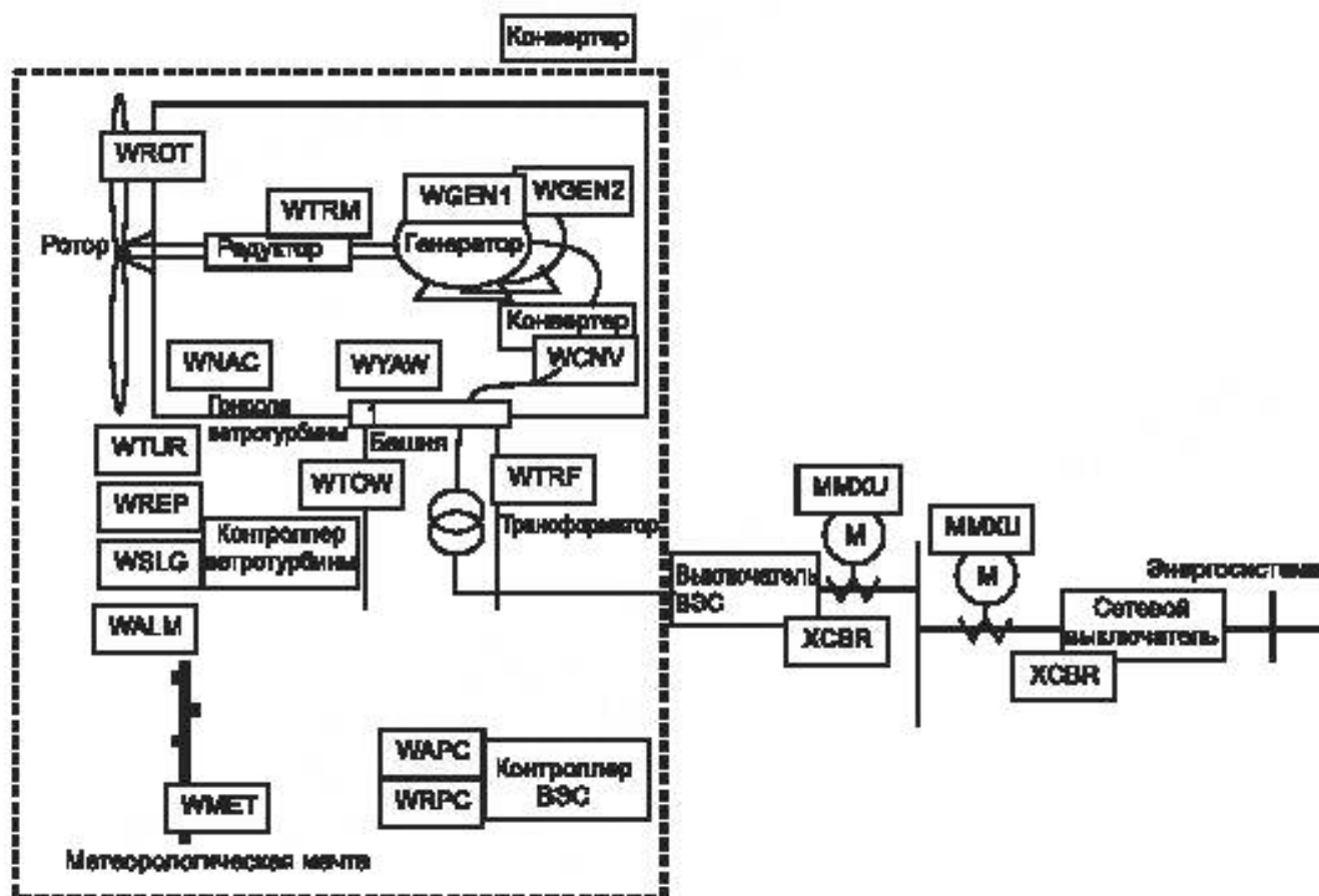
1 – Система ориентации по ветру Рисунок 3 – Использование логических узлов
