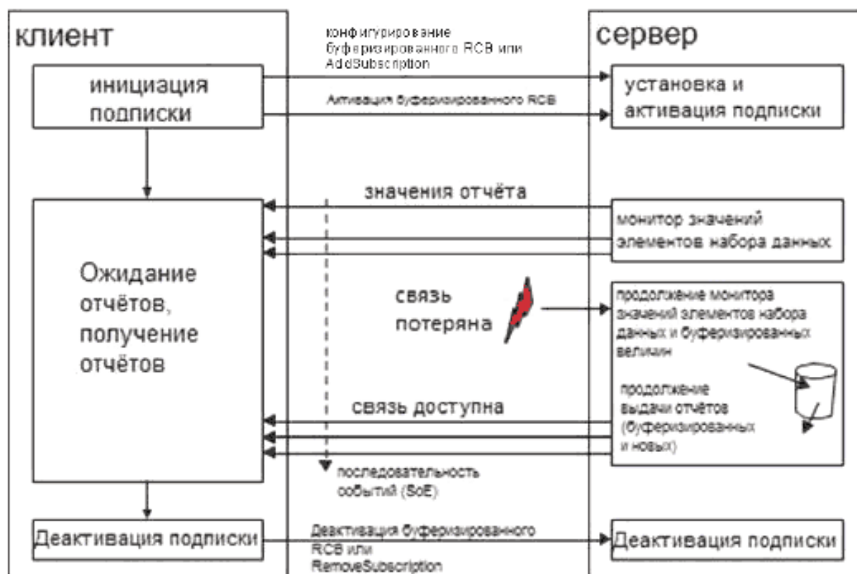
Рисунок 6 – Концепция блока управления буферизированным отчетом
