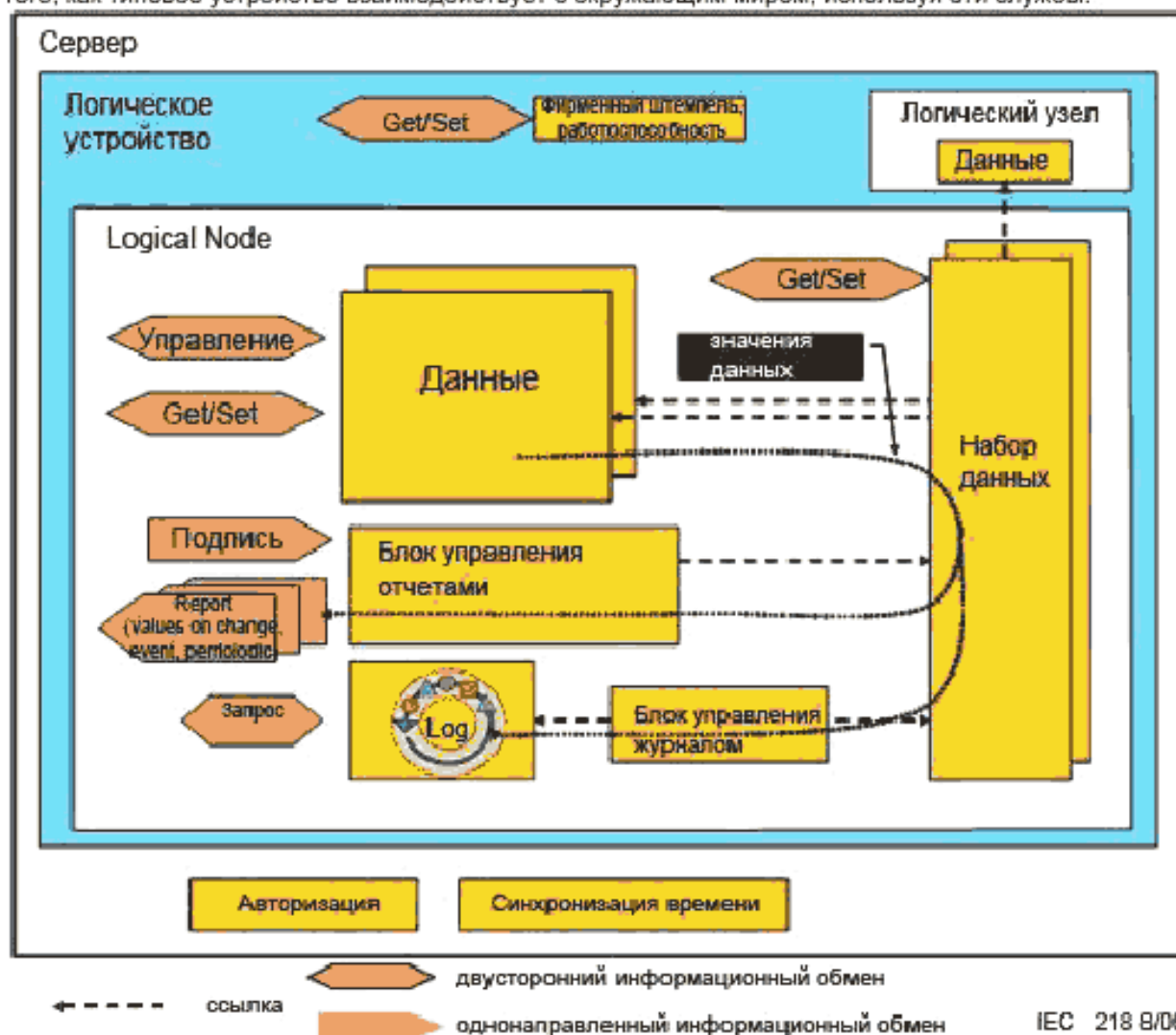
Рисунок 5 – Концепция модели обмена информацией ВЭУ
