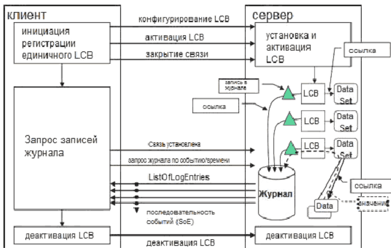
Рисунок 7 – Концепция блока управления журналом Log control block
