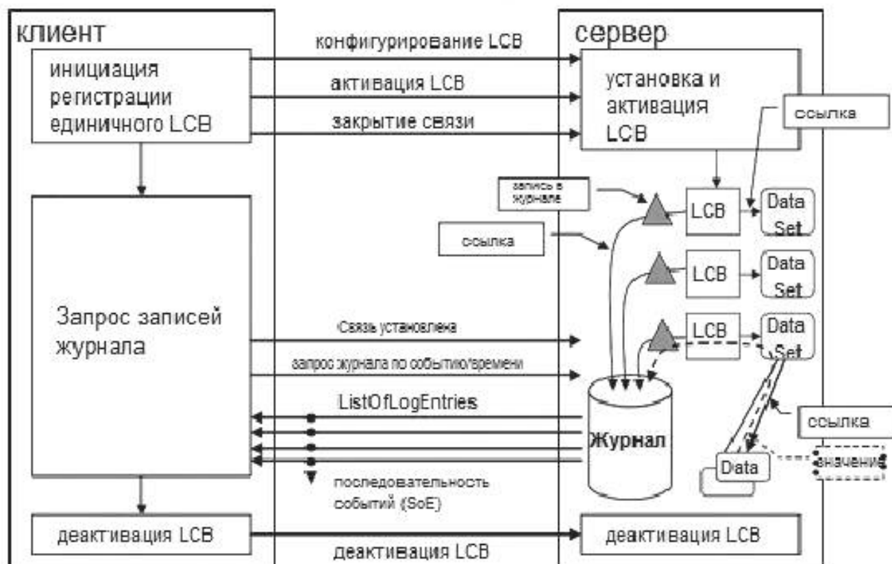
Рисунок 7 – Концепция блока управления журналом Log control block
