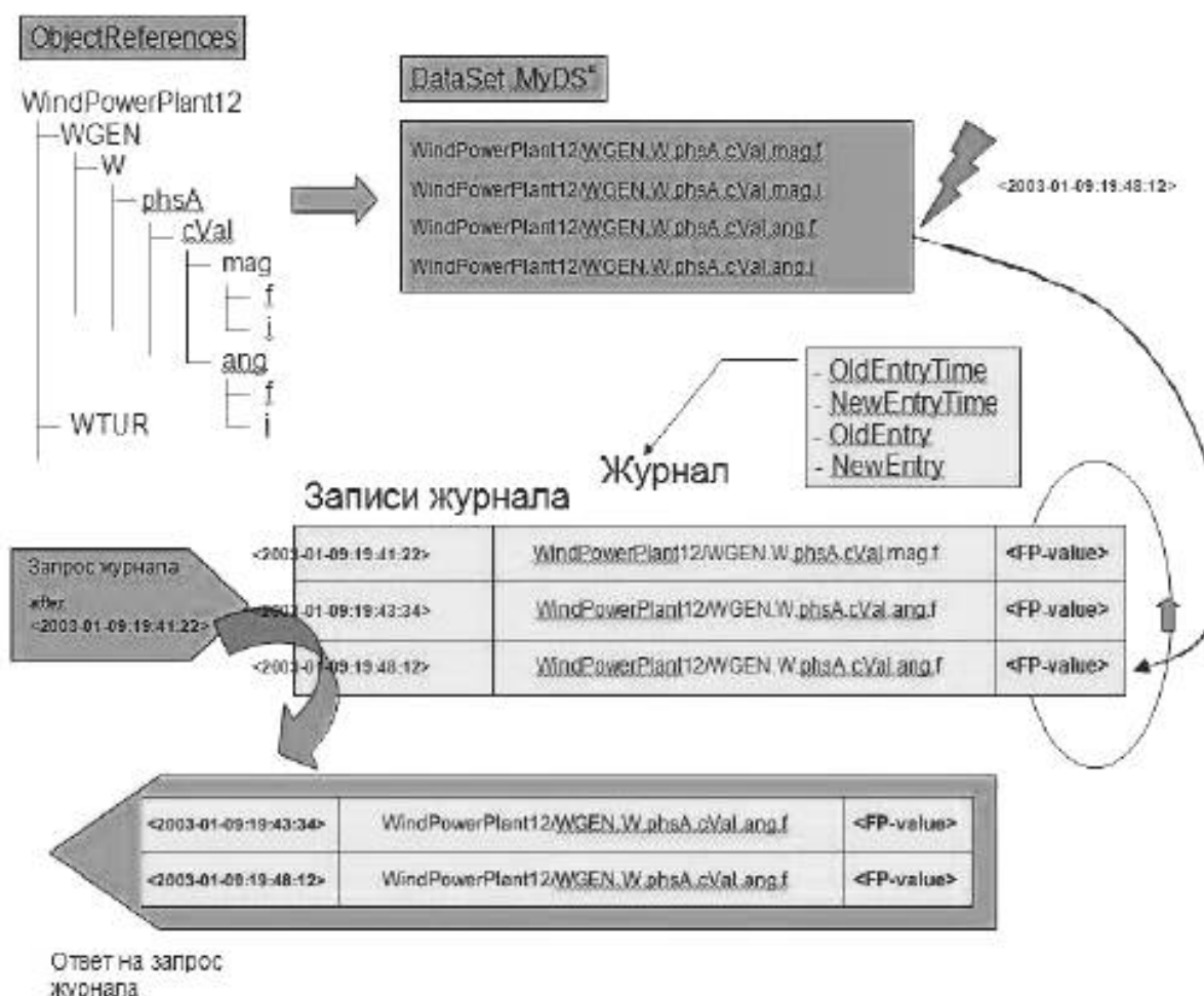
Рисунок А.2 – Основы регистрации (пример)
