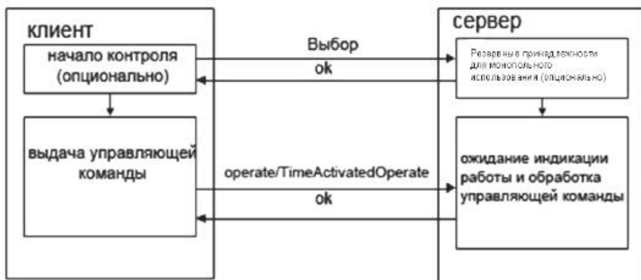
Рисунок 3 – Концепция модели управления
