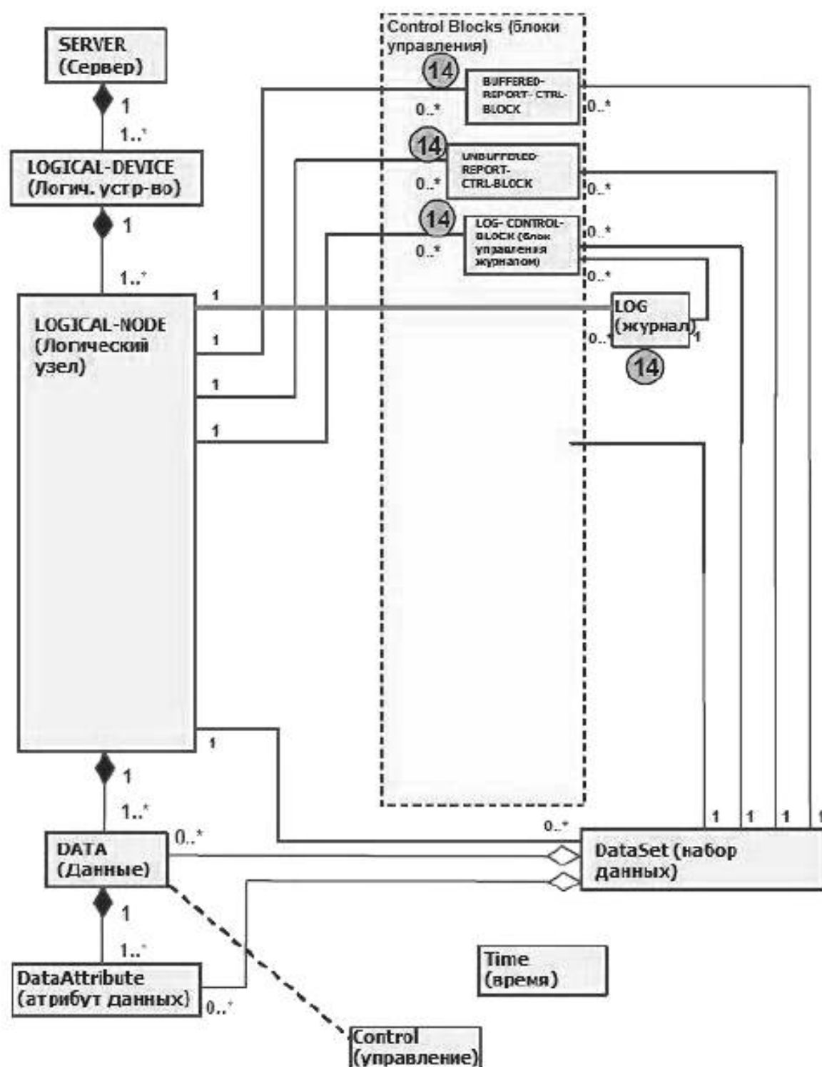
Рисунок В.1 – Концептуальная модель сервиса ACSI
