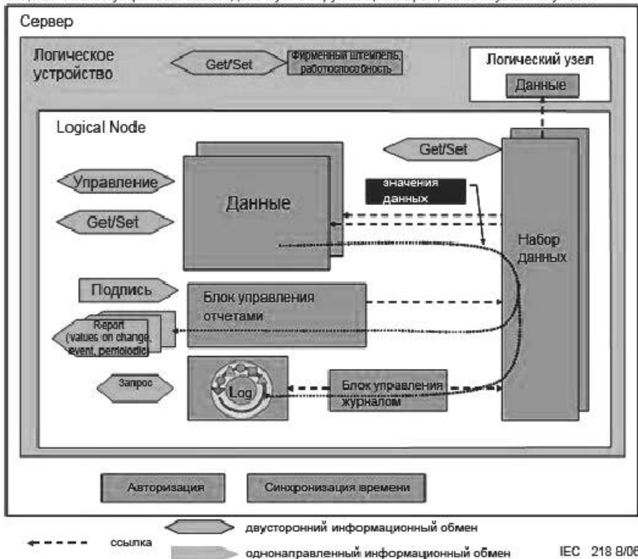
Рисунок 5 – Концепция модели обмена информацией ВЗУ
