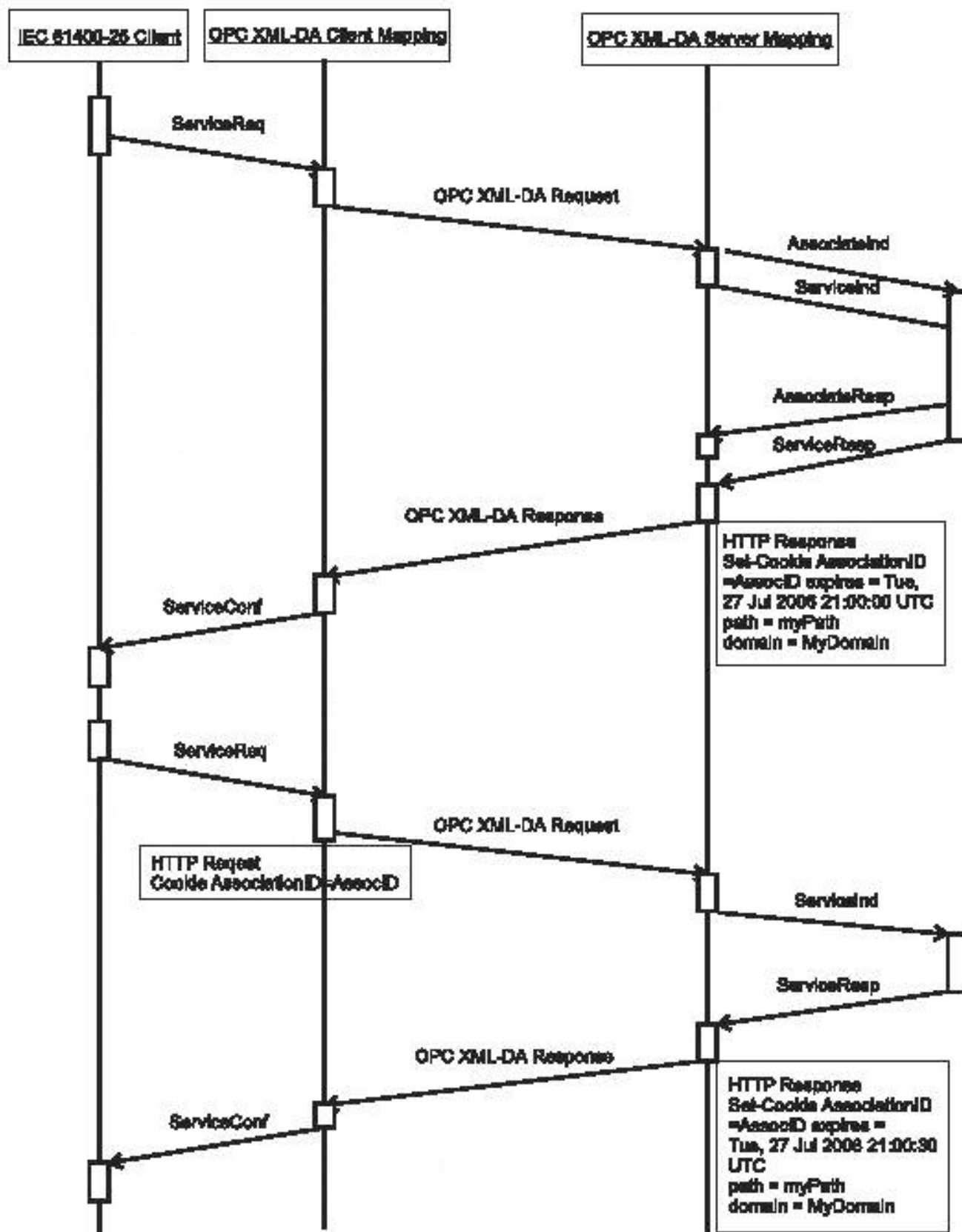
Рисунок Б.2 – Последовательность сервисов, устанавливающих ассоциацию
