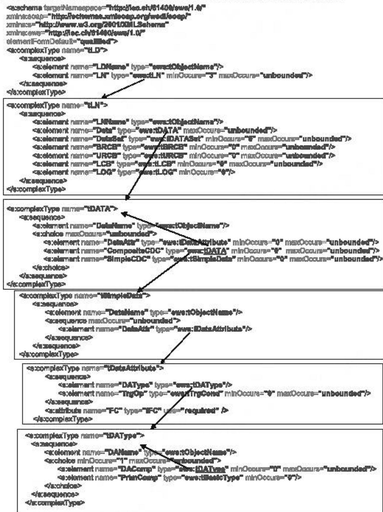
Рисунок A.2.1 – XML схема для информационной модели ВЗС
