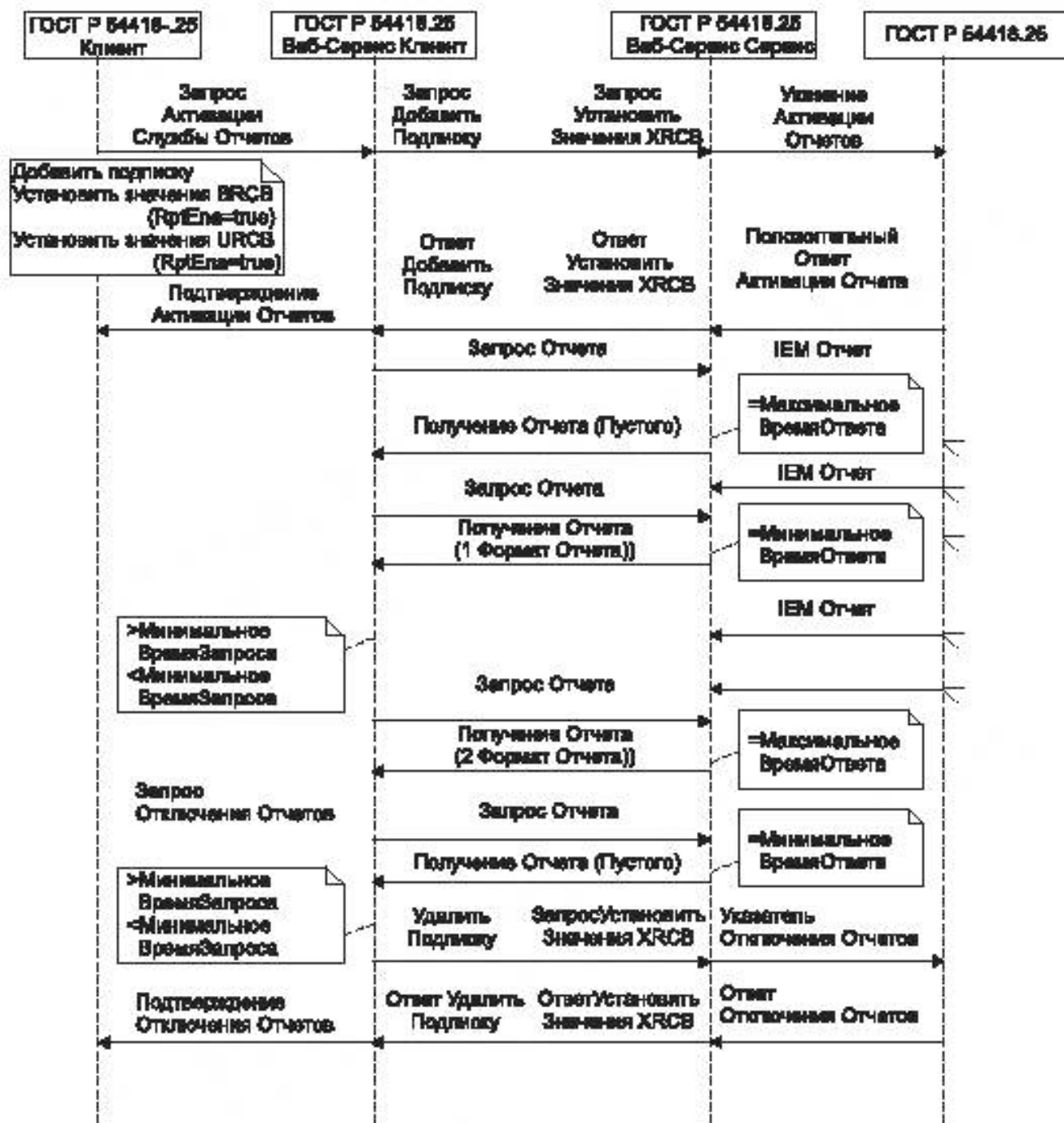
Рисунок А.5 – Механизм сервисов реализации отчетов (концепция)
