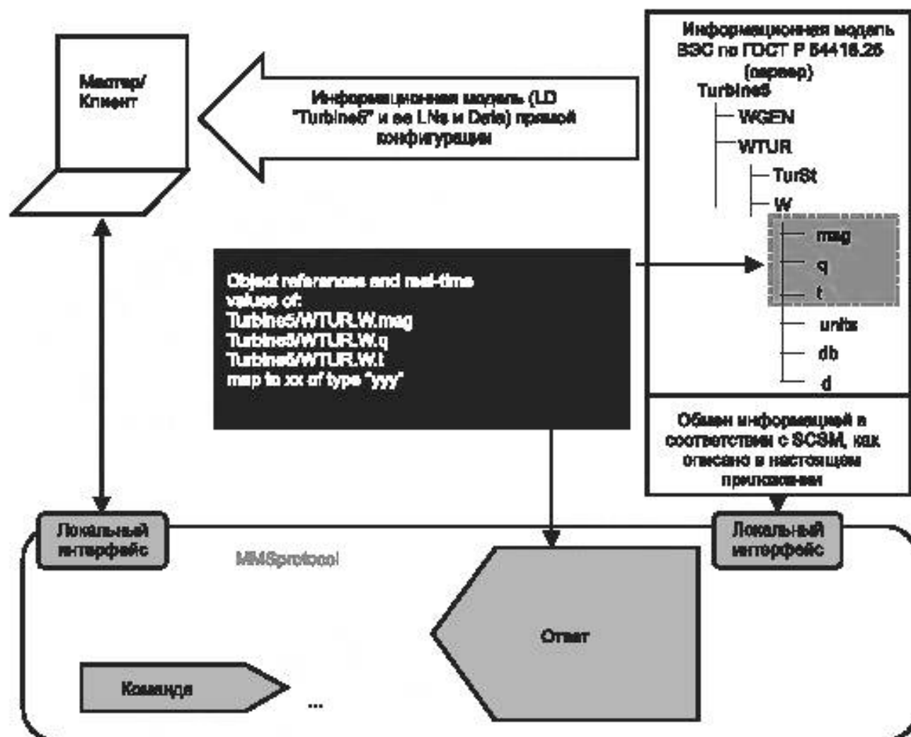
Рисунок В.1 – Архитектура отображения (схематическая)
