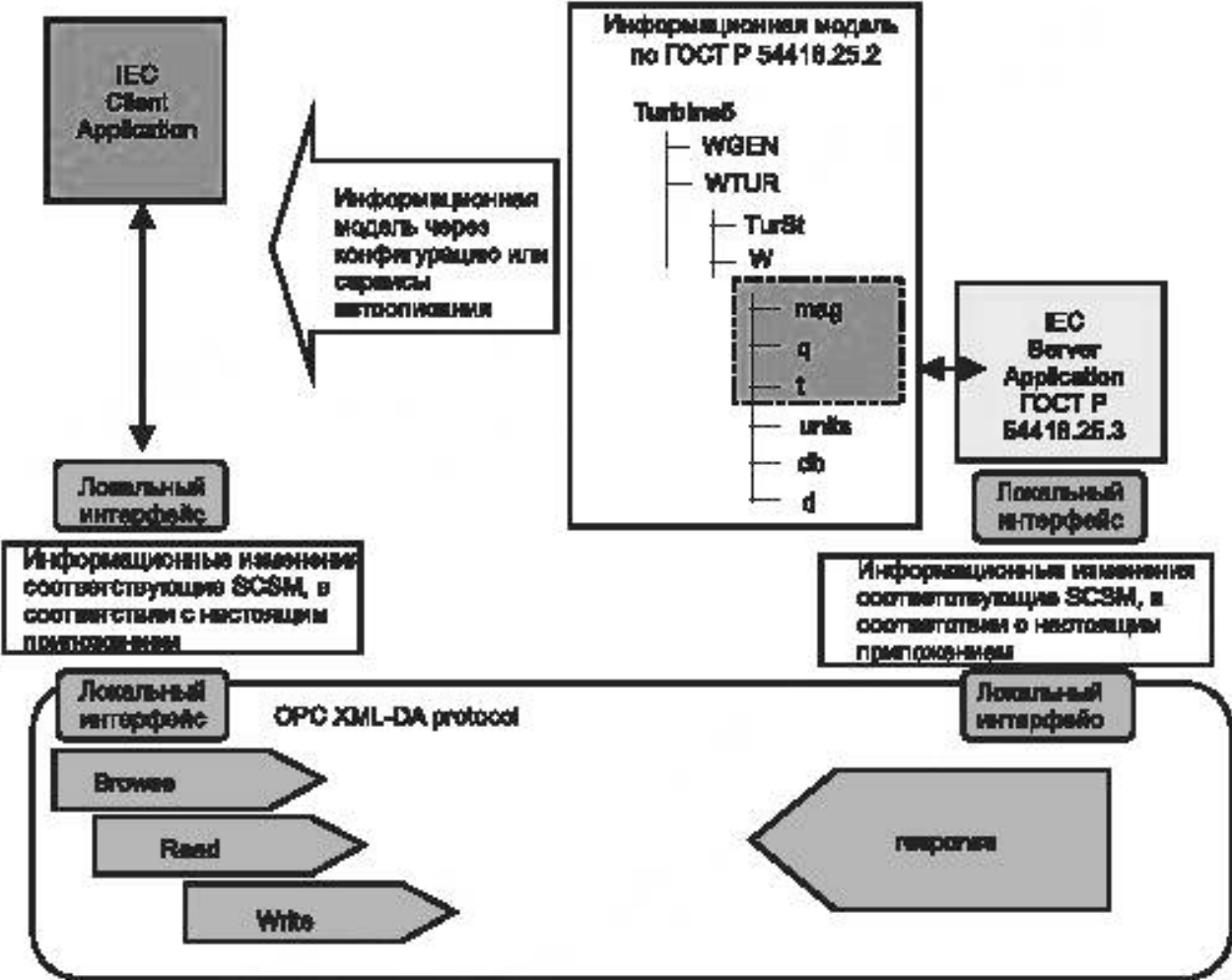
Рисунок Б.1 – Отображение (концептуальное) архитектуры
