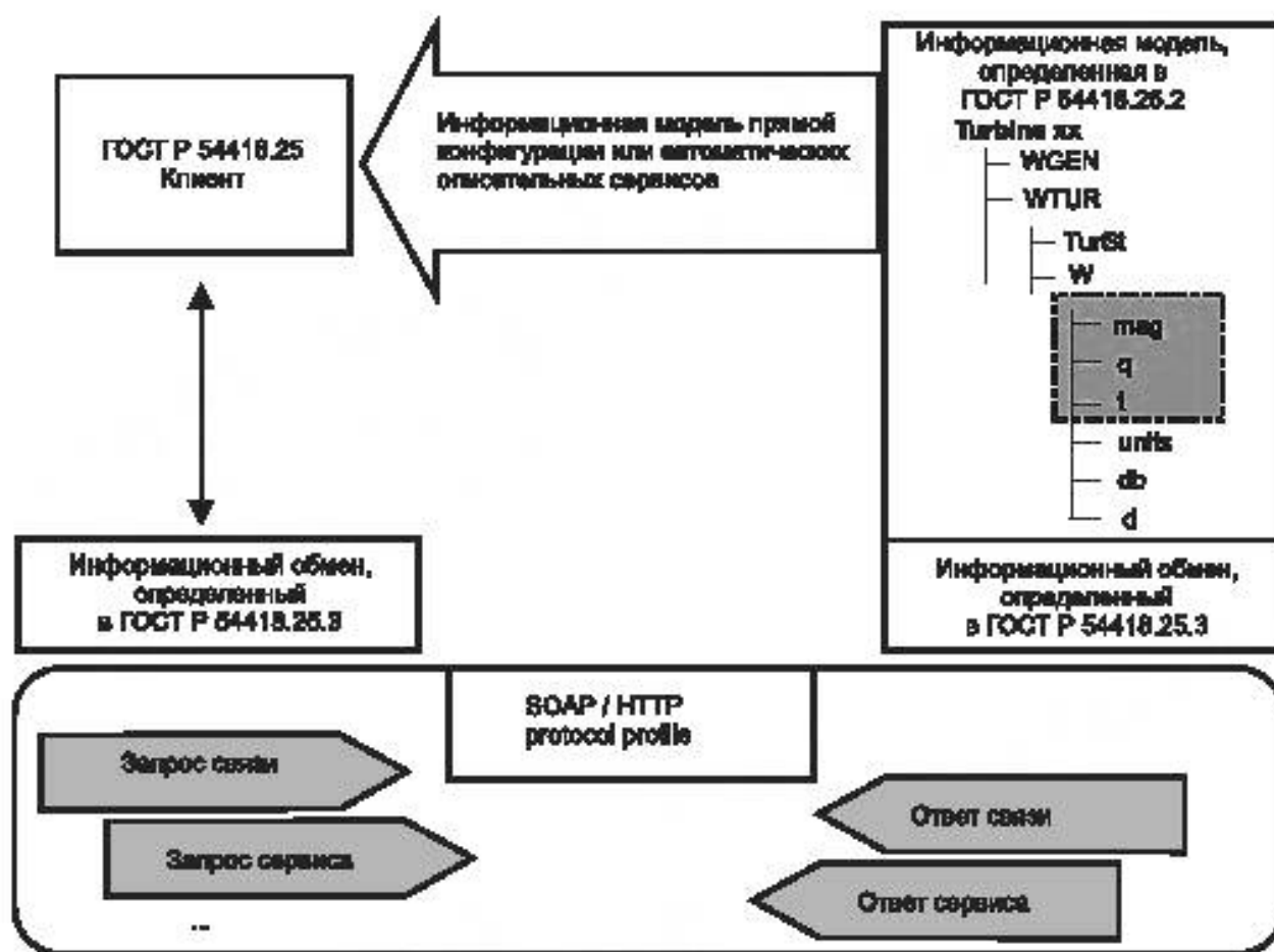
Рисунок А.1 – Структура отображения (концепция)
