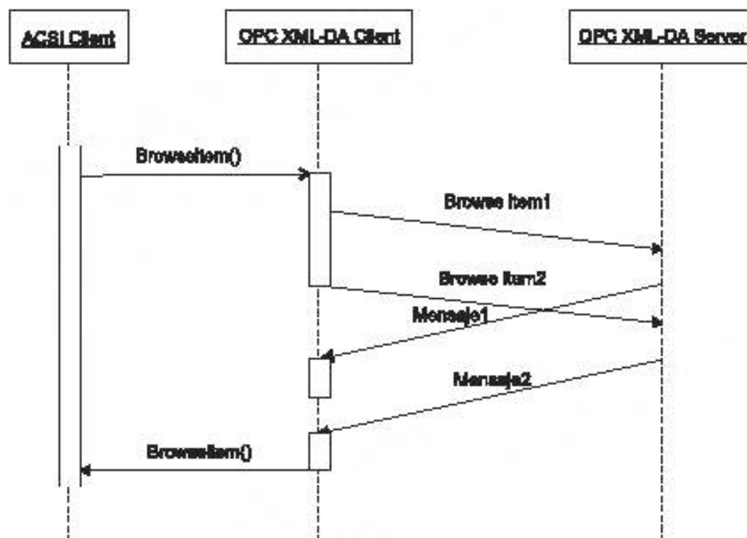
Рисунок Б.3 – последовательность сервисов CreateDataSet
