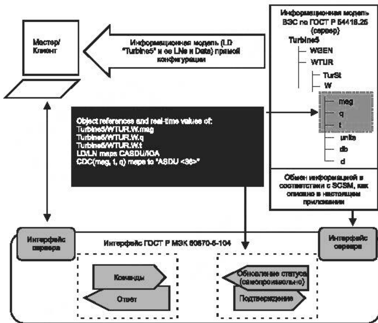
Рисунок Г.1 – Архитектура отображения (концептуальная)
