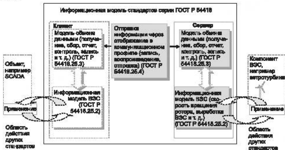
Рисунок 1 – Концептуальная коммуникационная модель серии стандартов ГОСТ Р 54418.25
