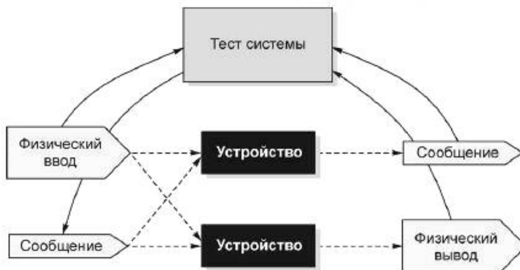
Рисунок 5 — Тестирование производительности (принцип черного квадрата)
