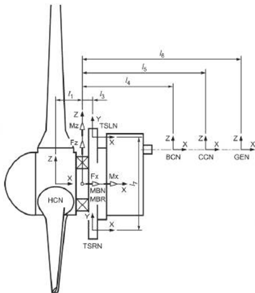
Рисунок 16 — Система координат в комплексной трансмиссии
