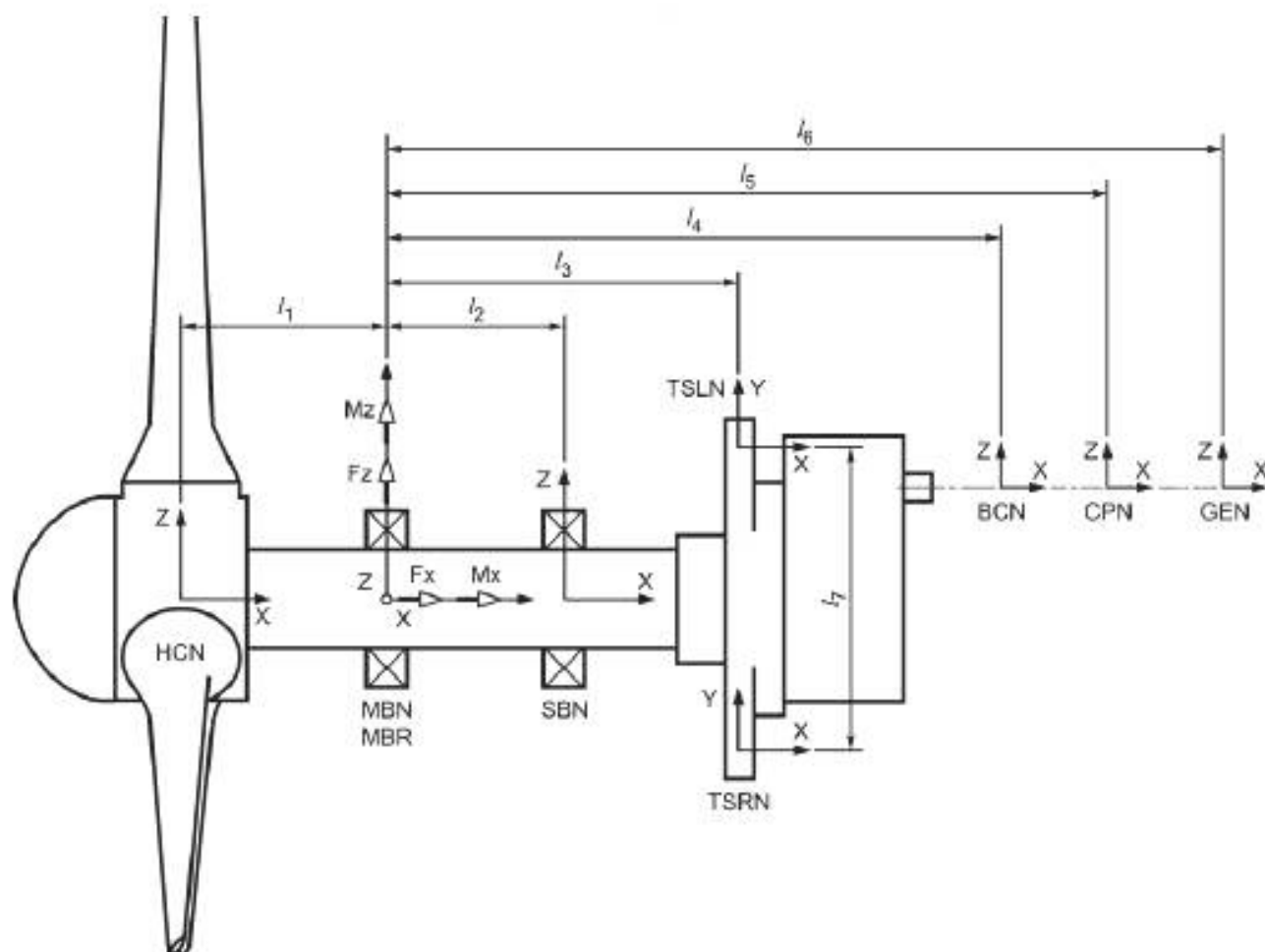
Рисунок 13 — Система координат в модульной трансмиссии
