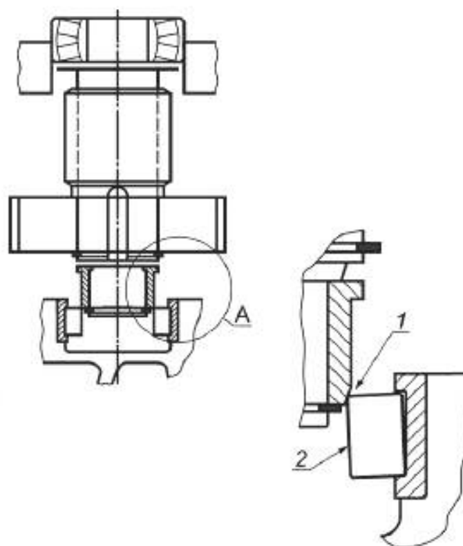
Вид А
