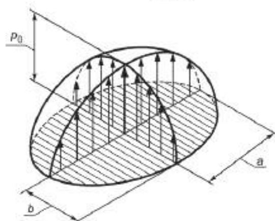
Рисунок 24 — Распределение напряжения по эллипсоидной контактной зоне
