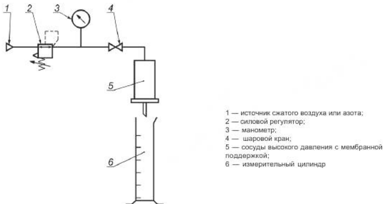
Рисунок 34 — Тестирование агрегата для оценки фильтрационной способности
