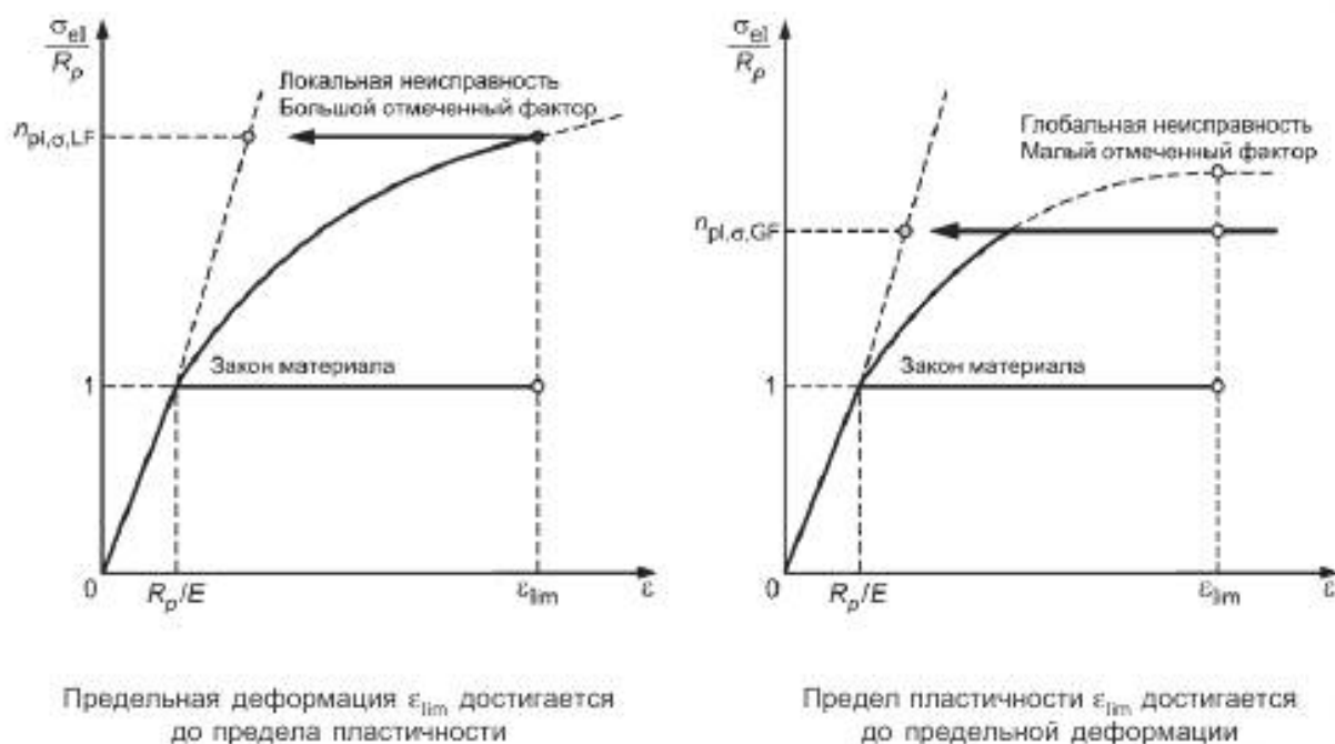
Рисунок 31 — Локальная и общая неисправности для двух разных радиусов пазов
