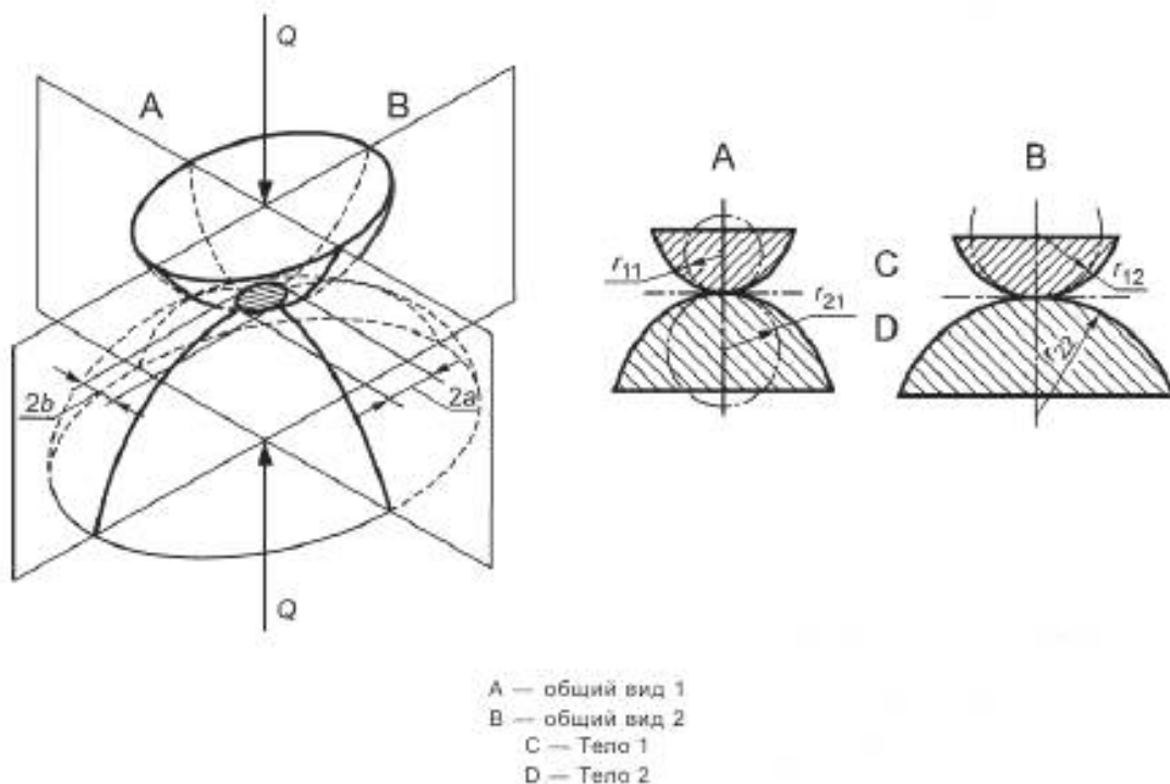
Рисунок 23 — Номенклатура кривых подшипника
