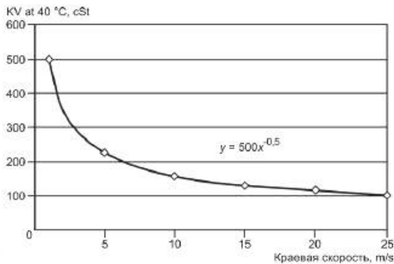
Рисунок 33 — Требования вязкости в зависимости от краевой скорости
