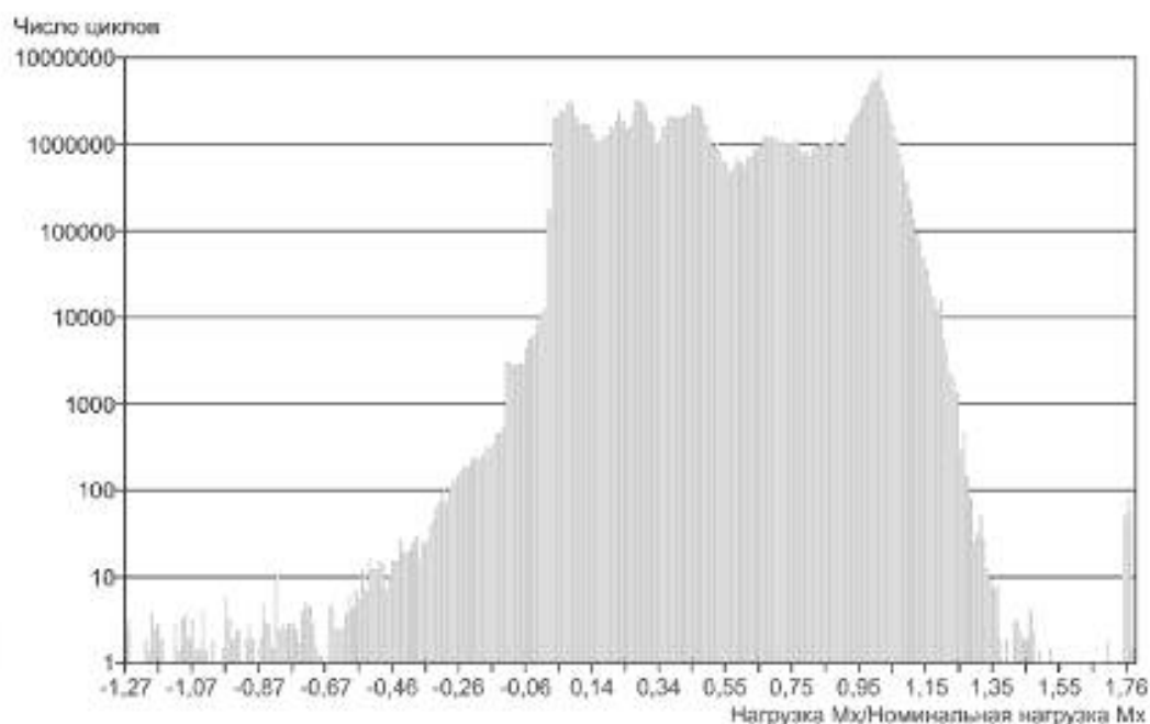
Рисунок 18 — Пример распределения нагрузки вращения (LRD)
