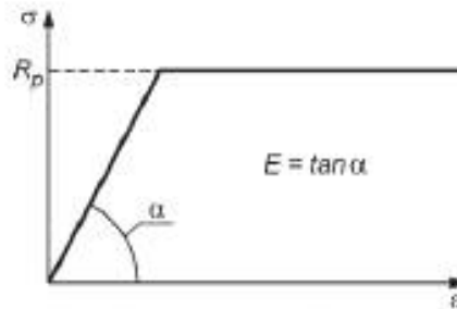
Рисунок 8 — Идеализированная зависимость упругой/пластичной деформации от напряжения
