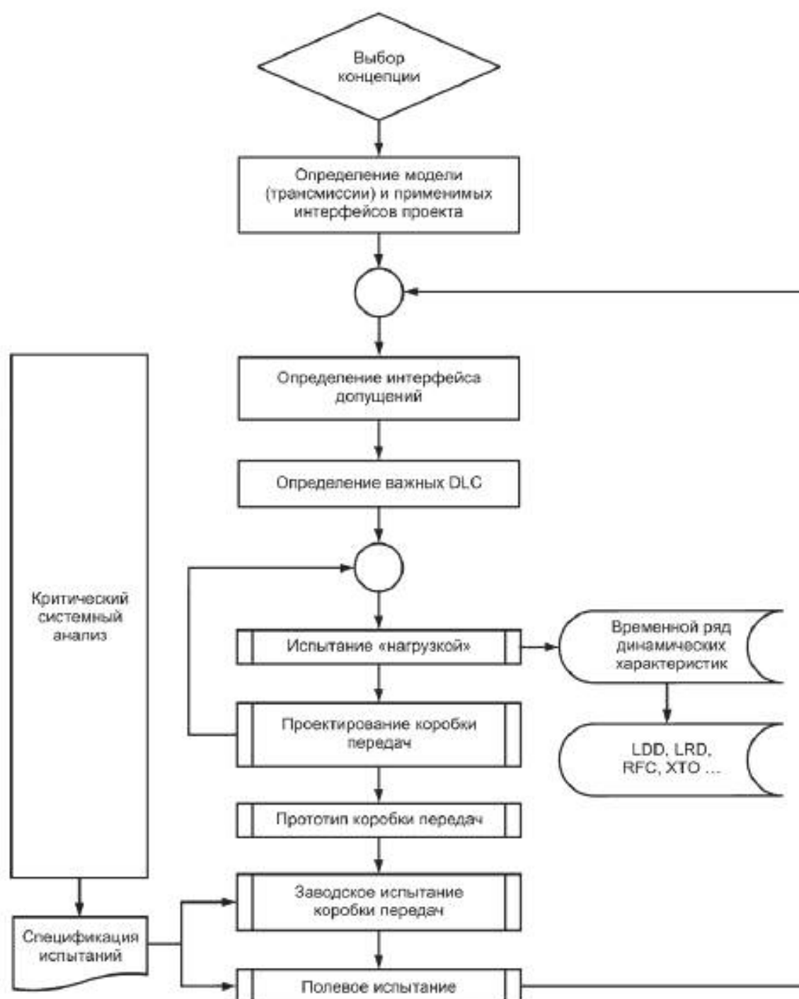
Рисунок 4 — Схема производственного процесса
