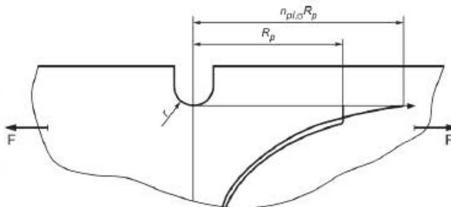
Рисунок 7 — Определение параметра секции n_{pl, \sigma} компонента с пазом
