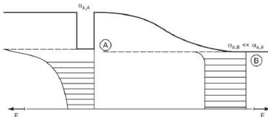
Рисунок 30 — Расположение локальной и общей неисправностей
