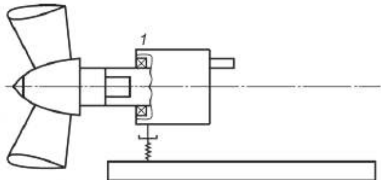
Рисунок 12 — Комплексная трансмиссия
