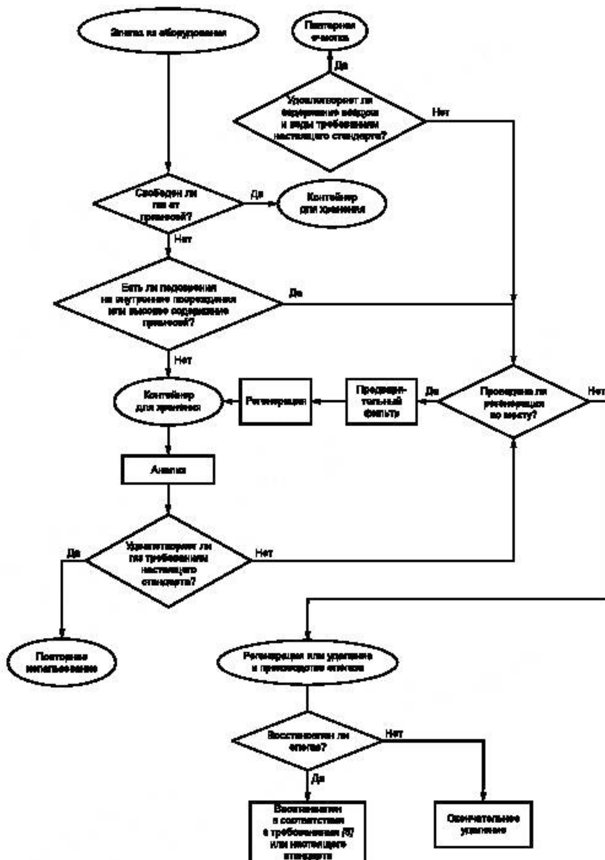
Рисунок 1 — Блок-схема для принятия решений по размещению или удалению элемента
