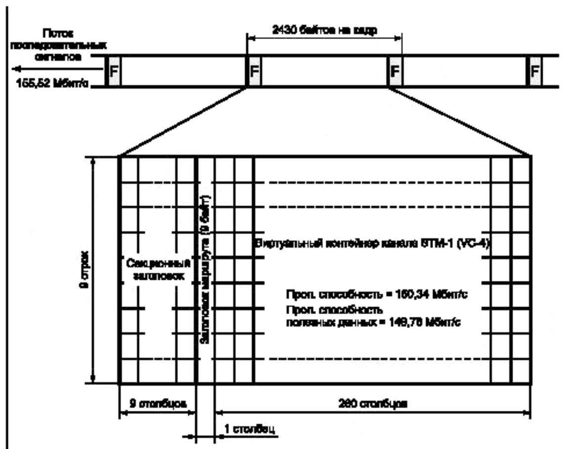
Рисунок 11 — Структура кадров канала STM-1
