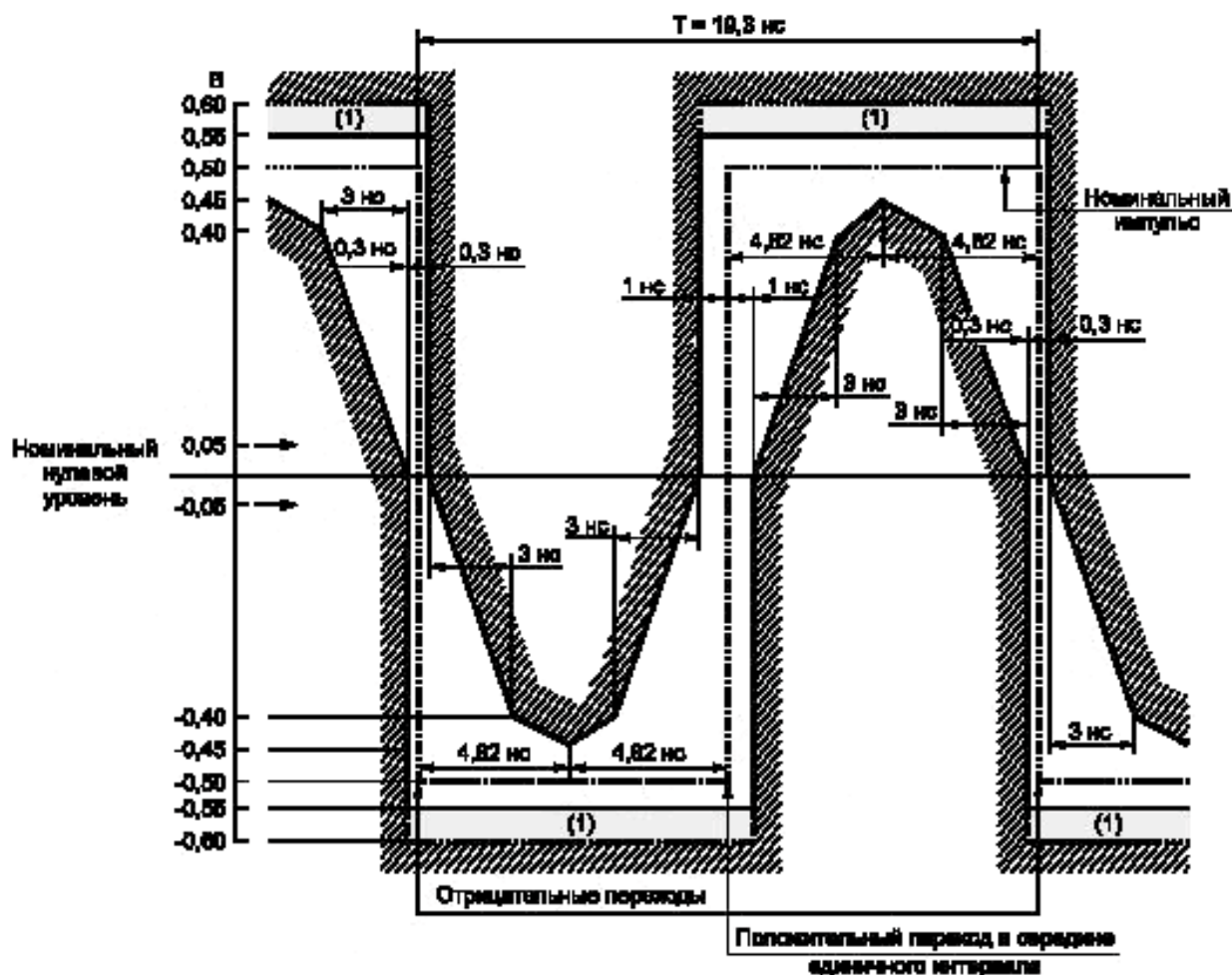
Рисунок Б.3 — Маска импульса 51840 кбит/с 1 (СМI; «0»)
