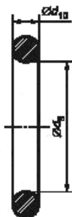
Рисунок ДА.3 — O-образные уплотнительные кольца
