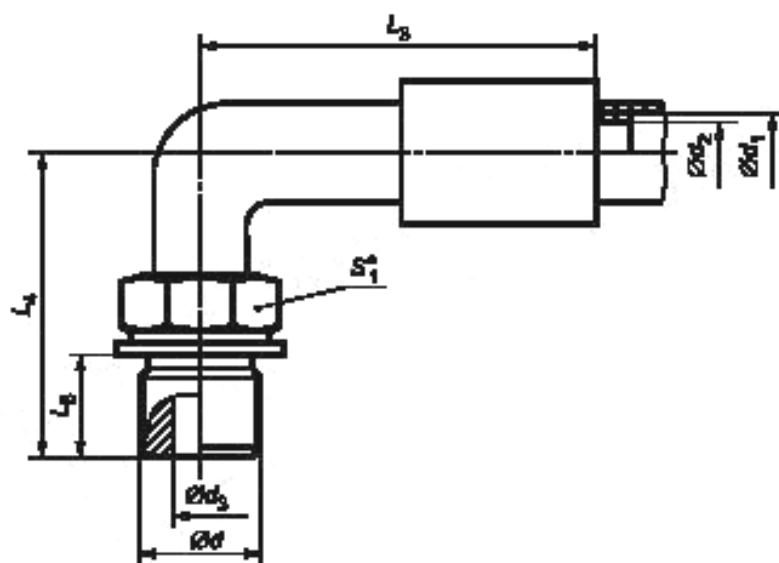
а) Угловой шланговый фитинг с углом изгиба 90^\circ (SDE) с метрическим ввертным концом, регулируемым по направлению, по приложению ДА (рисунок ДА.1)
