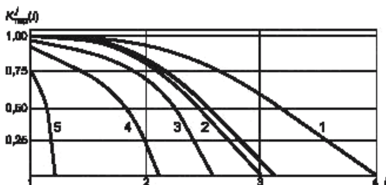
Рисунок 2 — Зависимость K(i) , нанесенная на серию тарифовочных кривых
