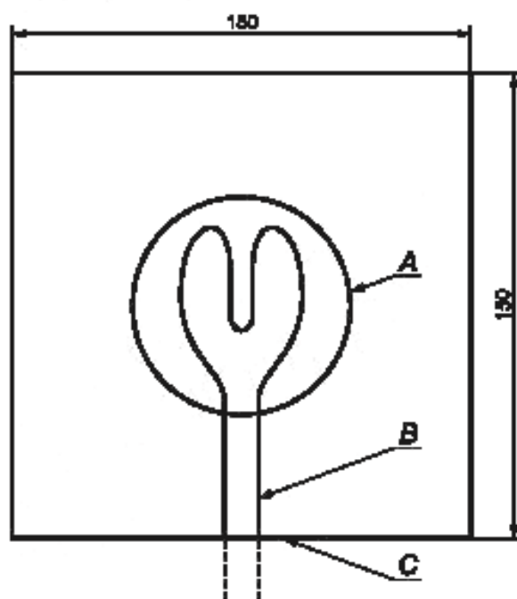
Рисунок 2 — Испытательная пластина и провод зажигания для проведения испытания окисляющей твердой химической продукции
