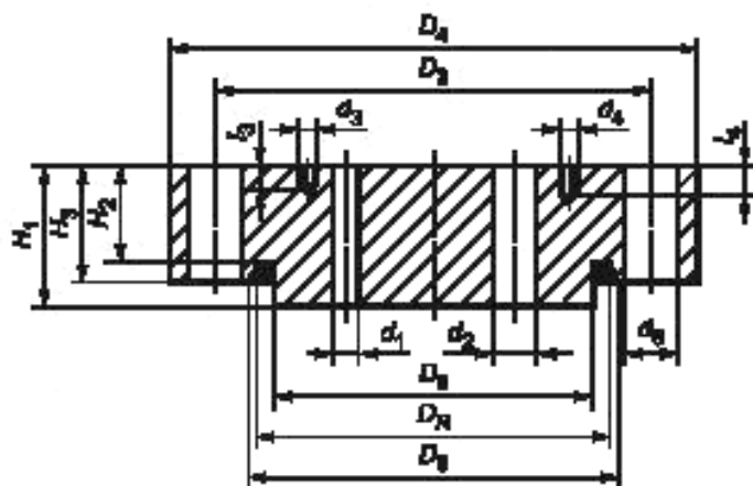
Рисунок 8.1 — Схема плоской крышки
