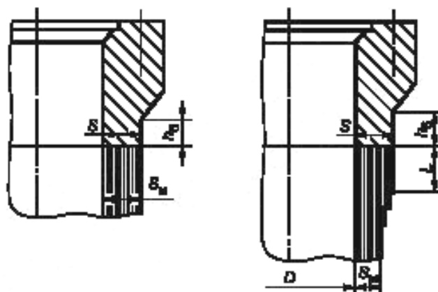
Рисунок 7.2 — Кованый фланец, сопряженный с многослойной обечайкой
