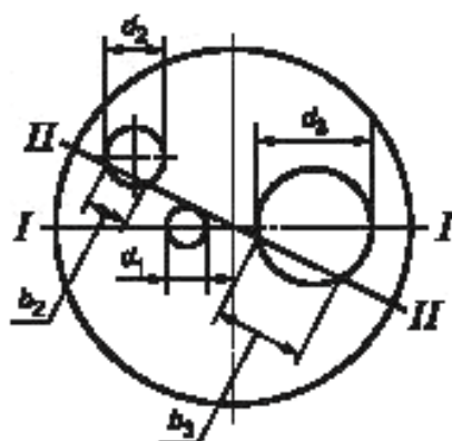
Рисунок 6.4 — Наиболее ослабленные диаметрально́е сечения днища
