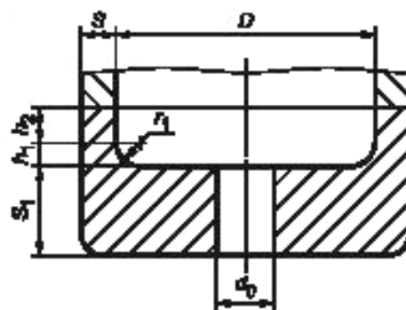
Рисунок 6.2 — Плоское днище с радиусным переходом
