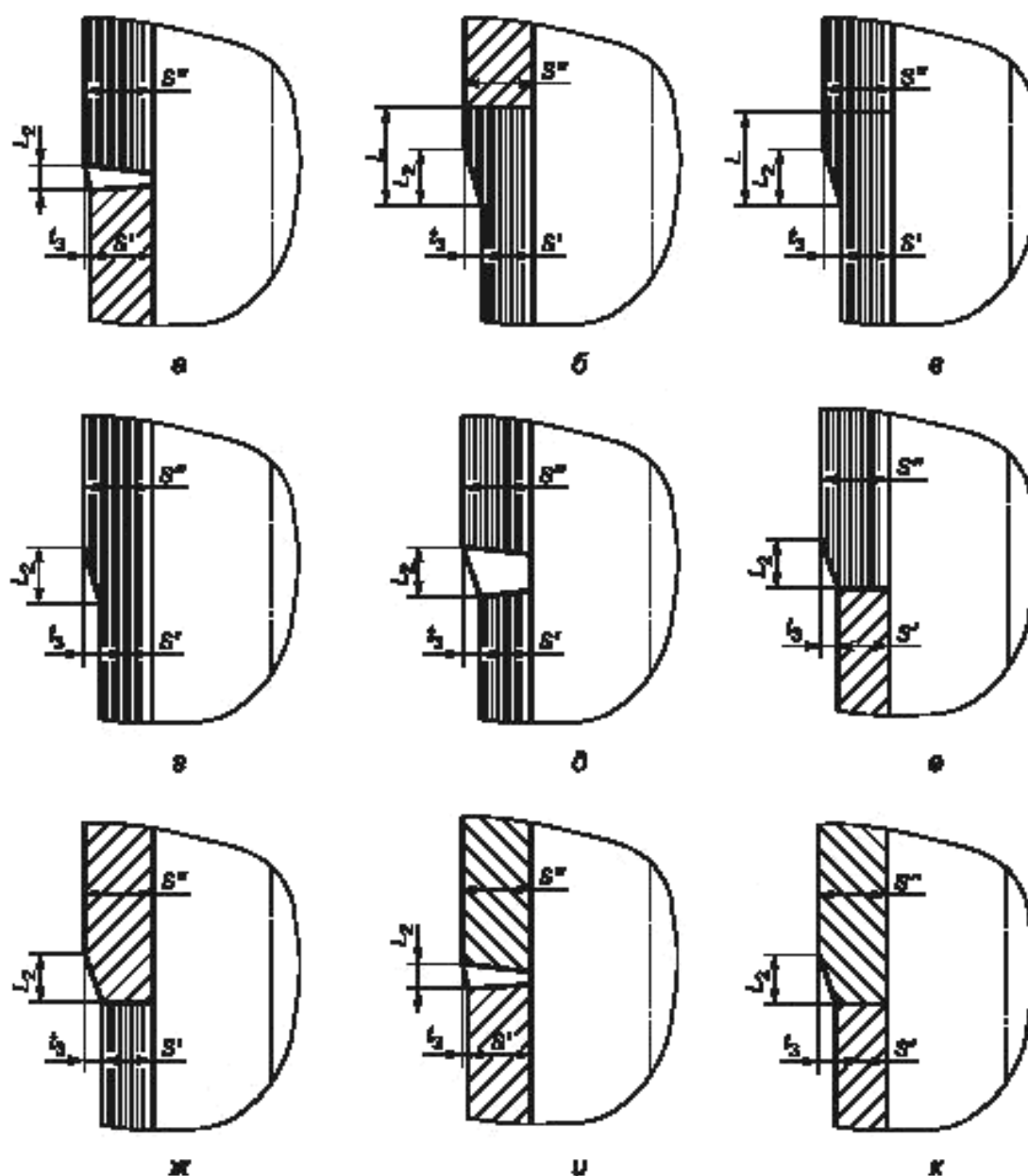
Рисунок 5.1 — Соединение цилиндрических обечаек
