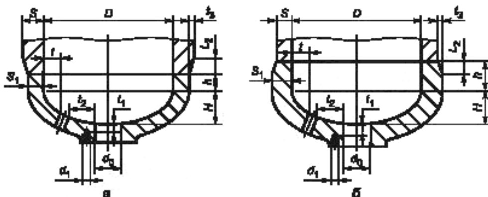
Рисунок 6.6 — Эллиптическое днище
