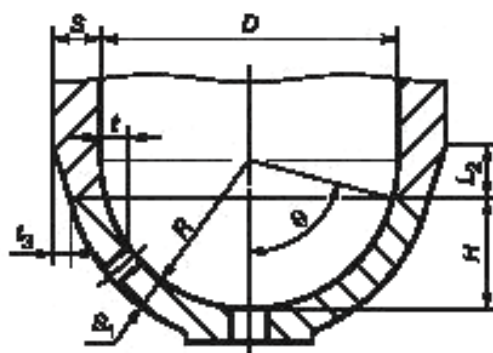
Рисунок 6.5 — Сферическое днище
