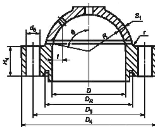
Рисунок 8.2 — Схема конструкции выпуклой крышки
