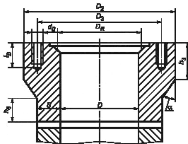
Рисунок 7.1 — Кованый фланец
