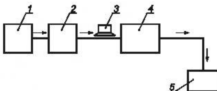
1 — компрессор; 2 — резервуар для стабилизации давления воздуха; 3 — маностат; 4 — центральное устройство (ротаметр); 5 — измерительная головка
