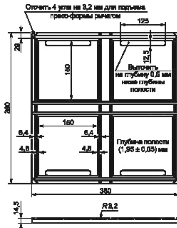
Рисунок 1 — Четырехполосная пресс-форма
