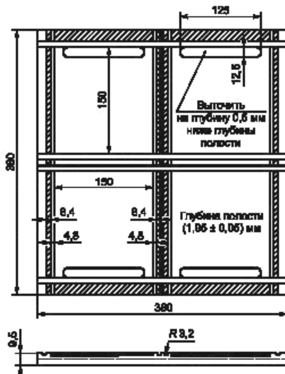
Рисунок 2 — Пресс-форма для гнезд, изготовленных в плите прессы
