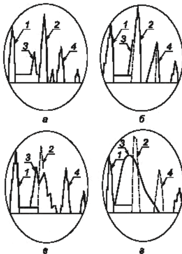
Рисунок В.1 — Вид эхо-сигналов на экране дефектоскопа
