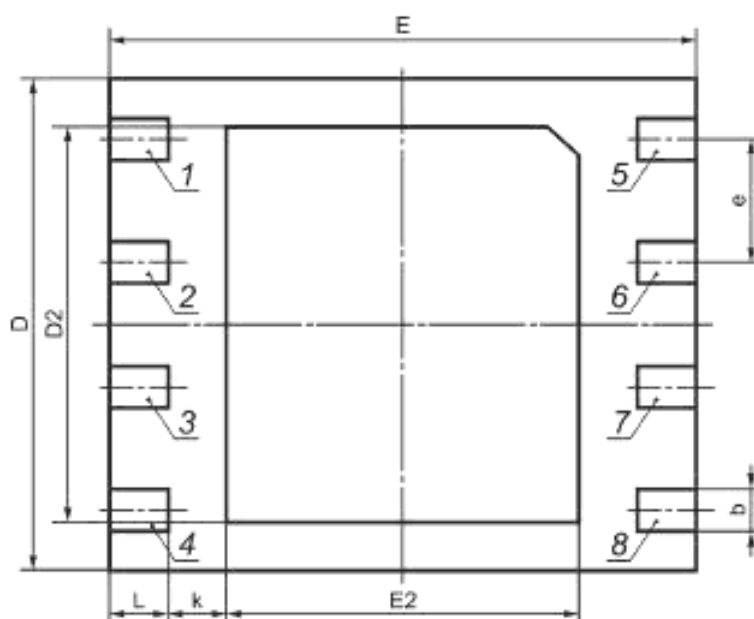
Рисунок 3 — Форм-фактор MFF2, вид снизу
