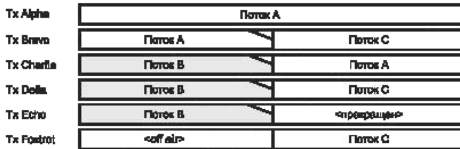
Рисунок Г.3 — Индивидуальные мультиплексные сообщения о реконфигурации FAC/SDC, создаваемые устройством MDI переключателя
