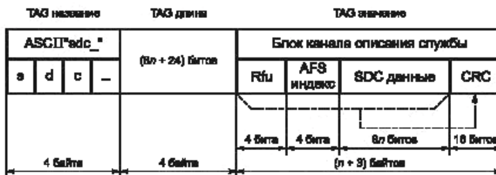
Рисунок 6 — Канал описания служб
