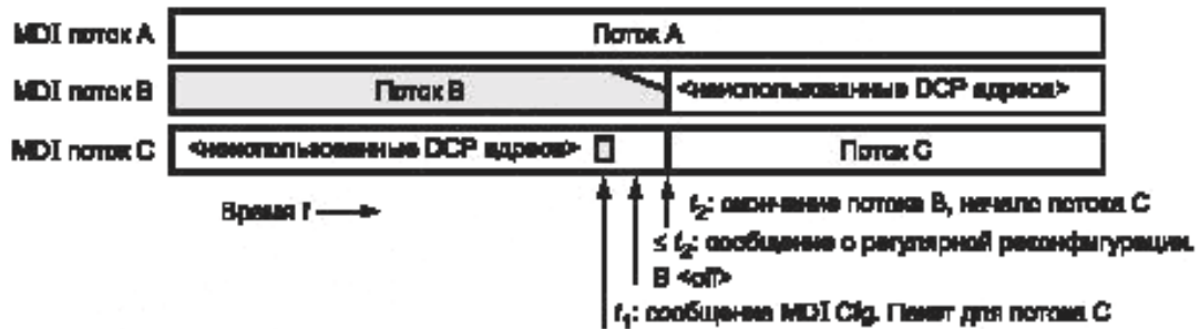
Рисунок Г.2 — Передача двух параллельных MDI потоков
