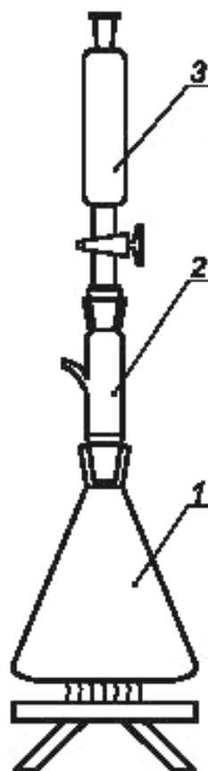
1 — колба Кн-1-500-29/32 ТС по ГОСТ 25336; 2 — переход П1О-29/32-14/23 ТС по ГОСТ 25336; 3 — воронка ВД-2-100 ХС по ГОСТ 25336
