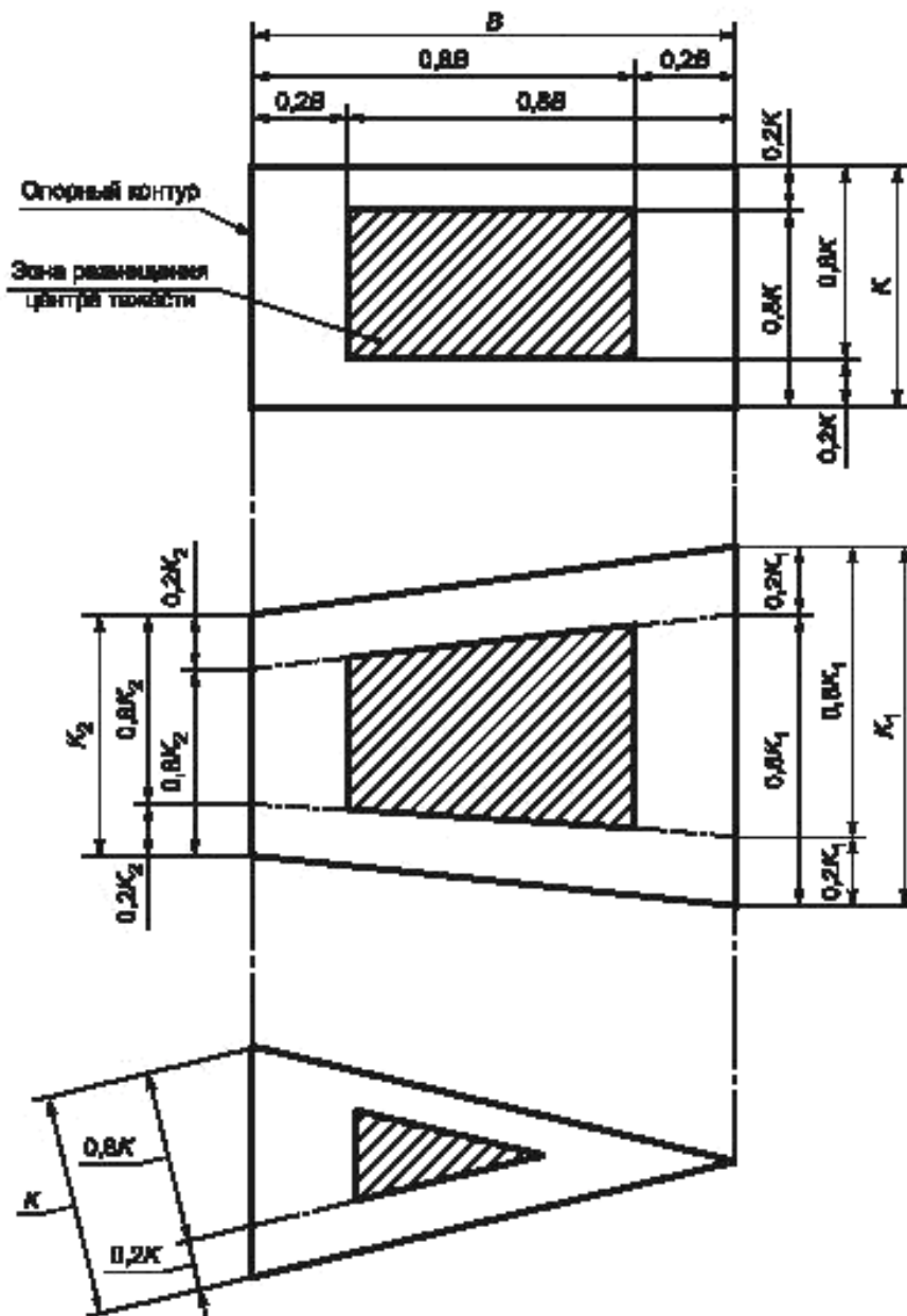
Рисунок 1 — Конфигурация основания грузоподъемного крана
