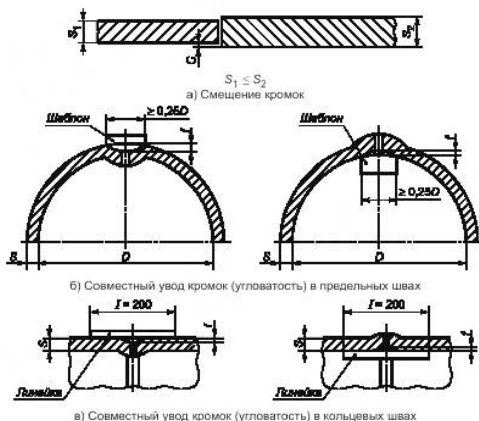
Рисунок 1 — Контроль смещения и увода кромок
