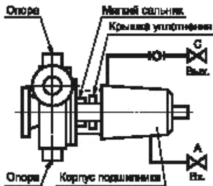
Схема А Охлаждение корпуса подшипника
