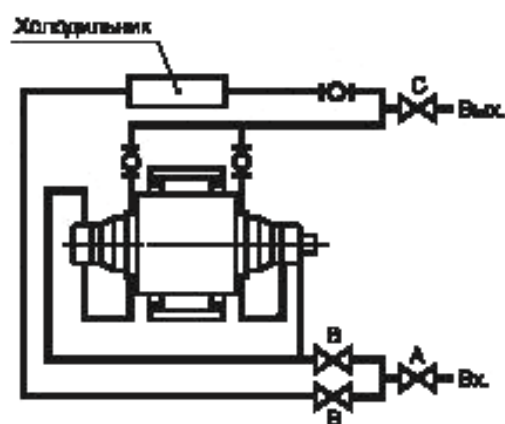
Схема K Последовательное охлаждение камеры мягкого сальника и корпуса подшипника с параллельной подачей в холодильник
