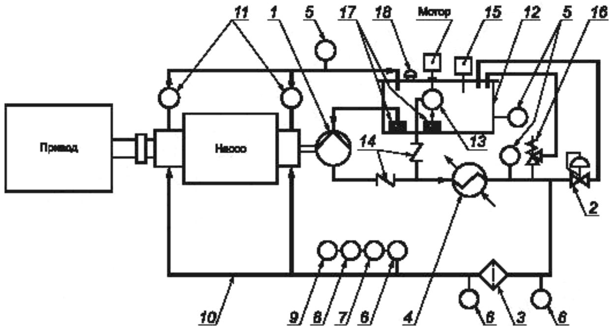
G.6 Типовая схема масляной смазки под давлением
