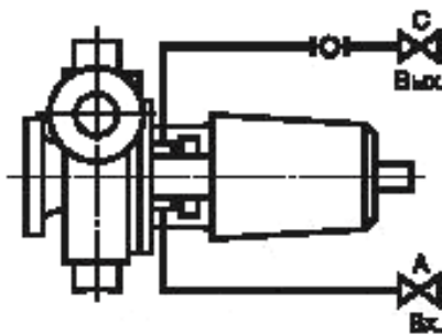
Схема С Охлаждение камеры мягкого сальника
