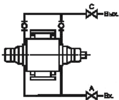
Схема С Охлаждение камеры мягкого сальника
