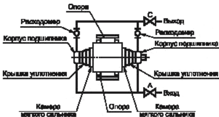
Схема А Охлаждение корпуса подшипника
