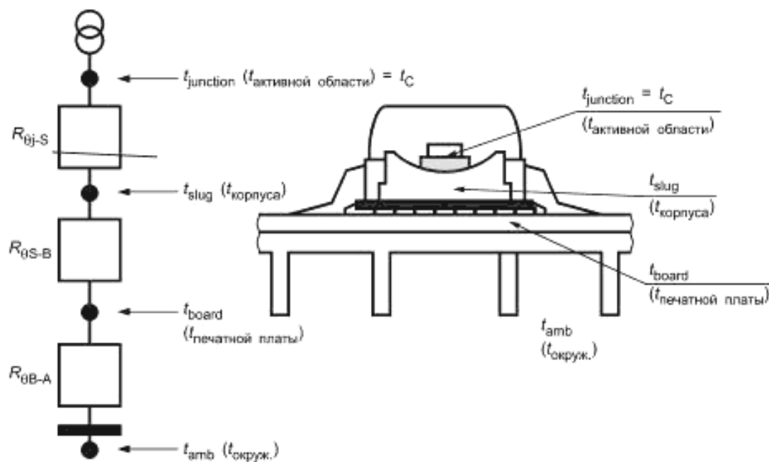
Рисунок 1 — Схематическая цепочка тепловых сопротивлений
