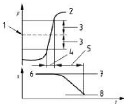
1 — регулируемое значение для давления срабатывания; 2 — контролируемое давление; 3 — AG; 4 — t < 0.2 с; 5 — время срабатывания t ; 6 — кривая закрытия; 7 — открыто; 8 — закрыто.
