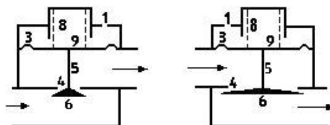
б) Тип 2. Регуляторы, нагруженные усилием пружины
