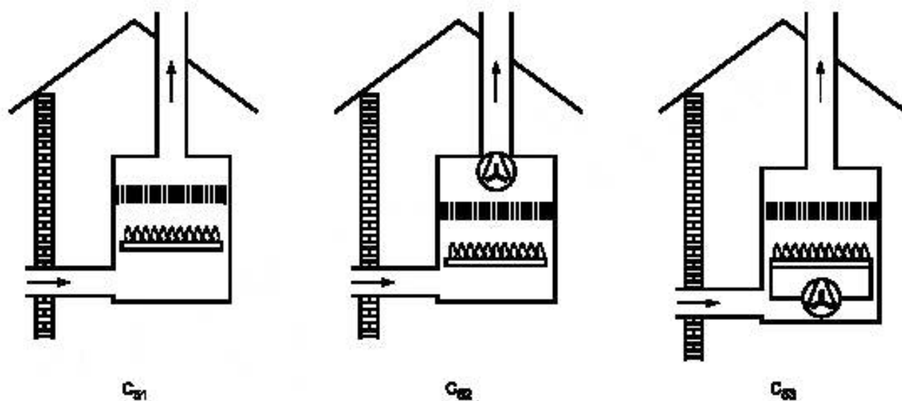
Рисунок В.5 — Схемы котлов типа C_5
