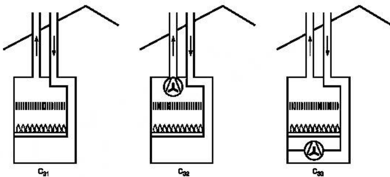
Рисунок В.3 — Схемы котлов типа C_3
