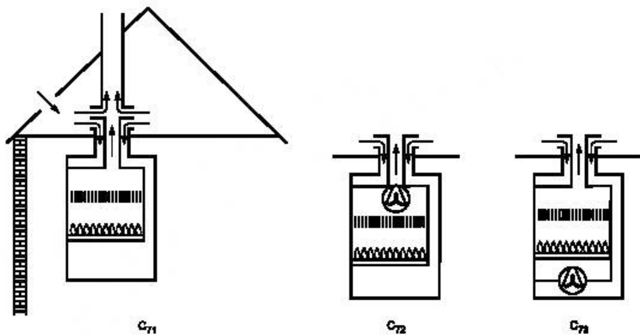
Рисунок В.7 — Схемы котлов типа C_7
