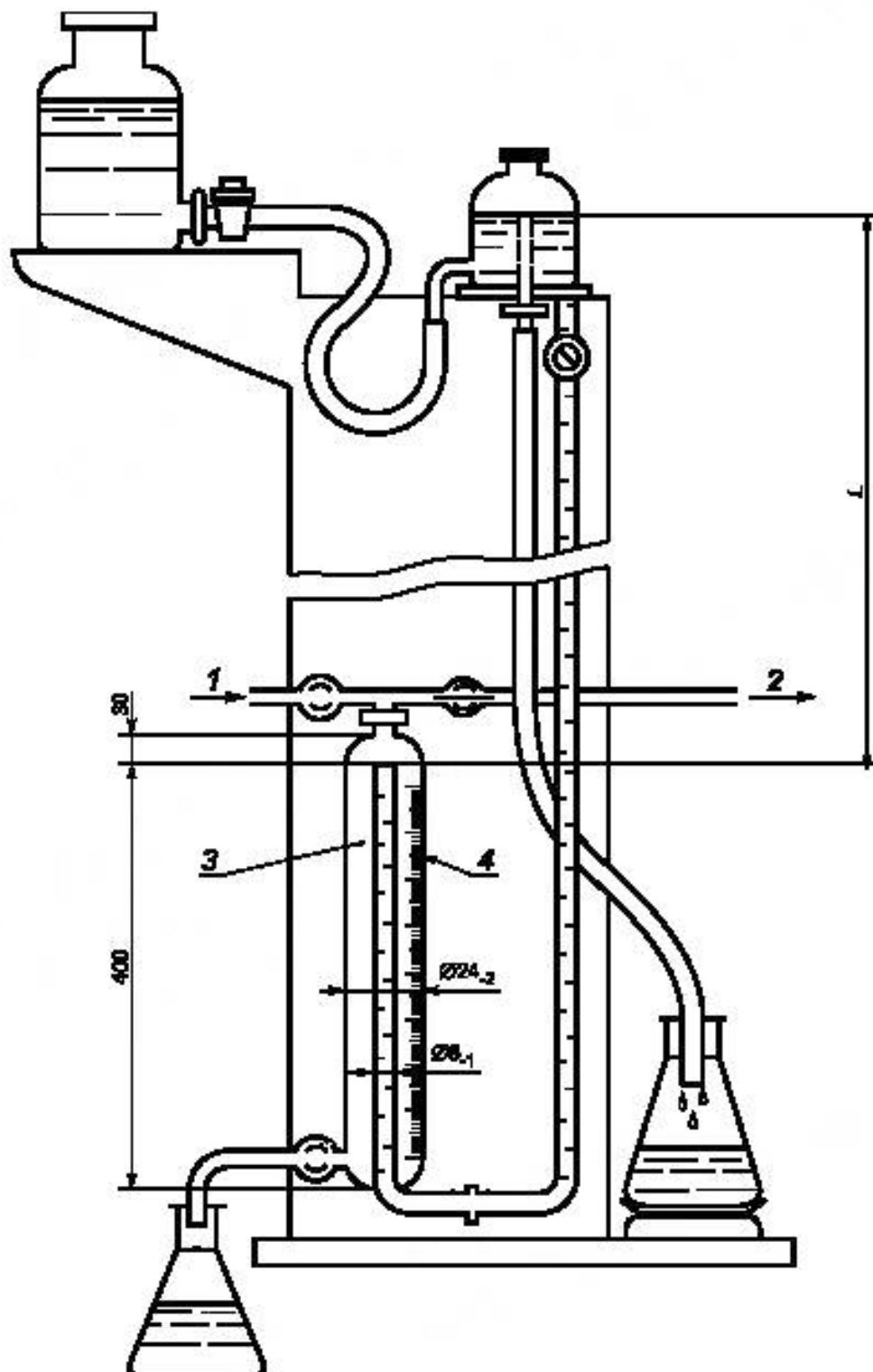
Рисунок 5 — Устройство для проверки герметичности газового тракта
