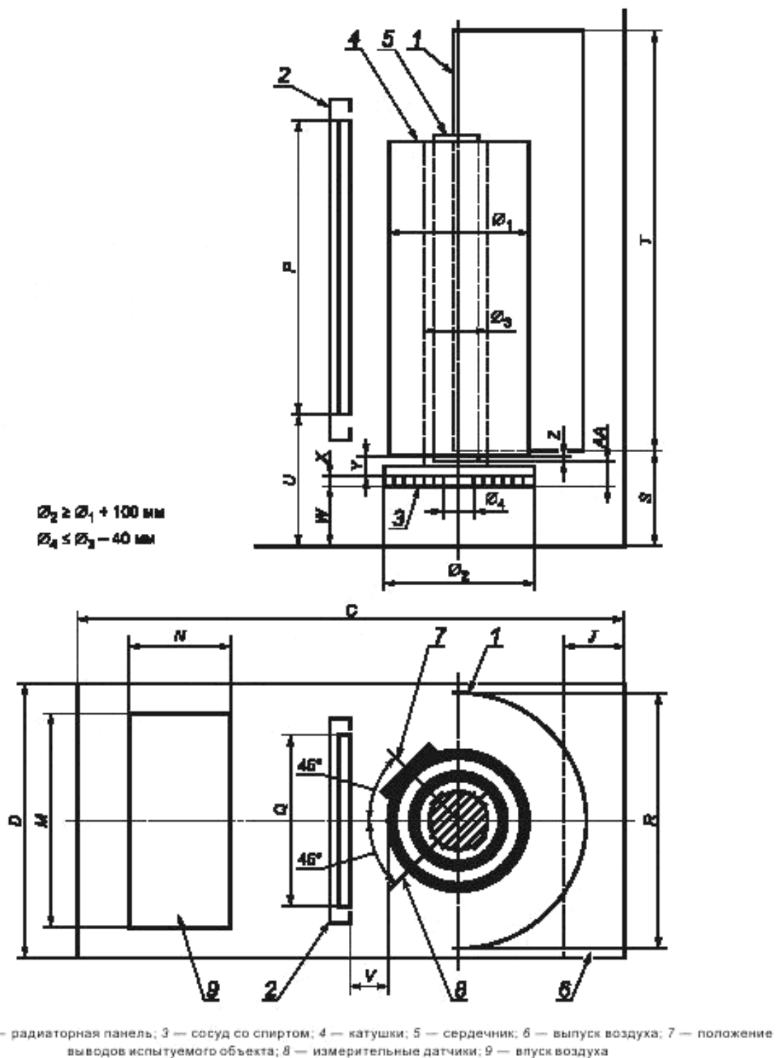
Рисунок 6 — Детали испытательной камеры
