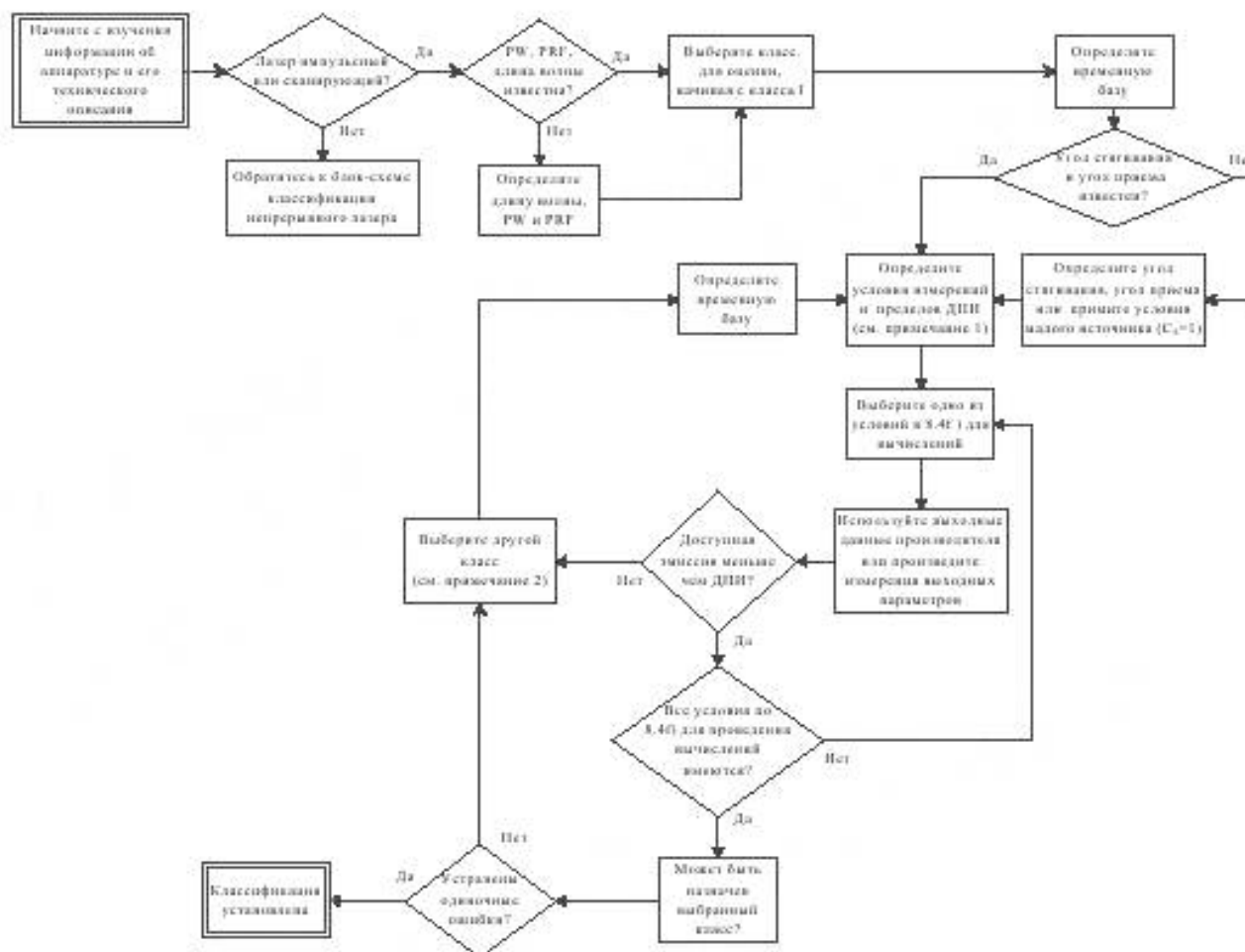
Рисунок 2 – Порядок проведения классификации импульсных лазеров
