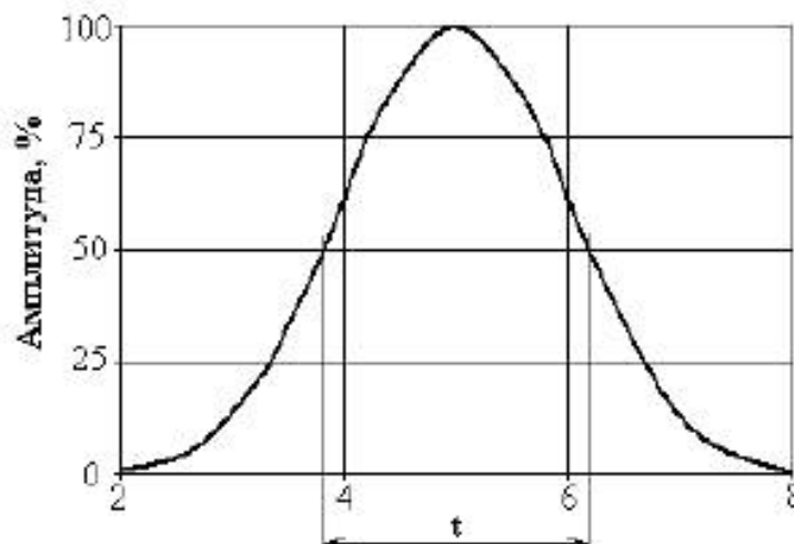
Рисунок 4 – Определение длительности импульса
