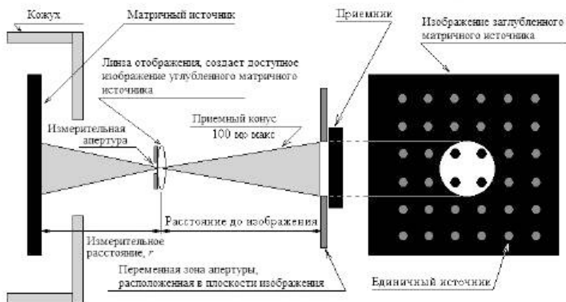
Рисунок 8b – Геометрия измерения для углубленного источника
