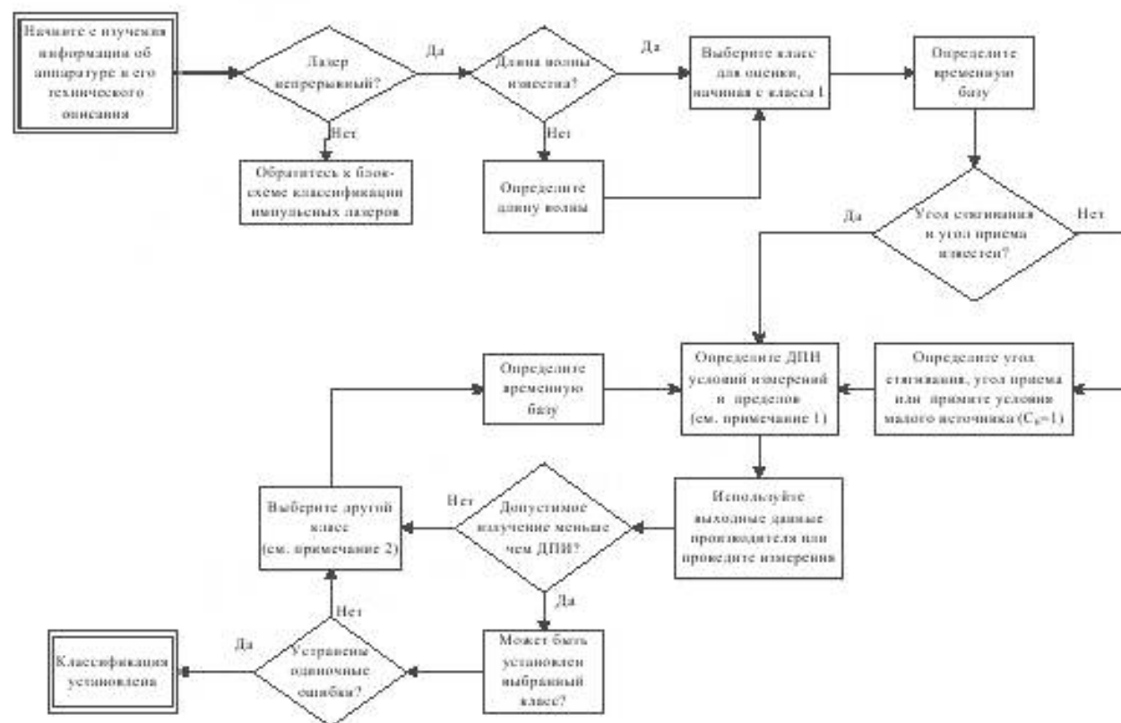
Рисунок 1 – Порядок проведения классификации лазеров непрерывного излучения
