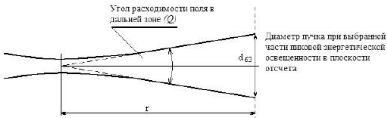
Рисунок 7 – Расположение перетяжки гауссовского пучка
