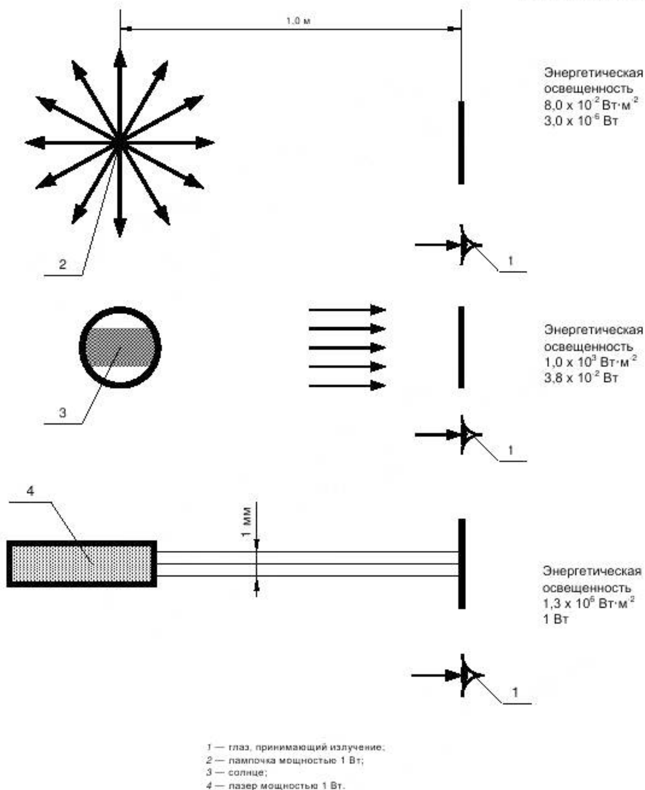
Рисунок 1 — Сравнение опасностей от различных источников света
