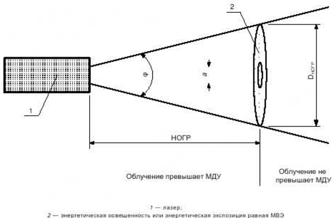
Рисунок 6 — Понятие номинального опасного для глаз расстояния
