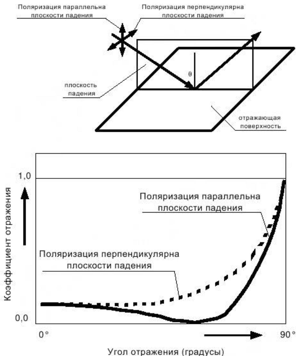
Рисунок 9 — Зеркальные отражения от поверхности прозрачных веществ
