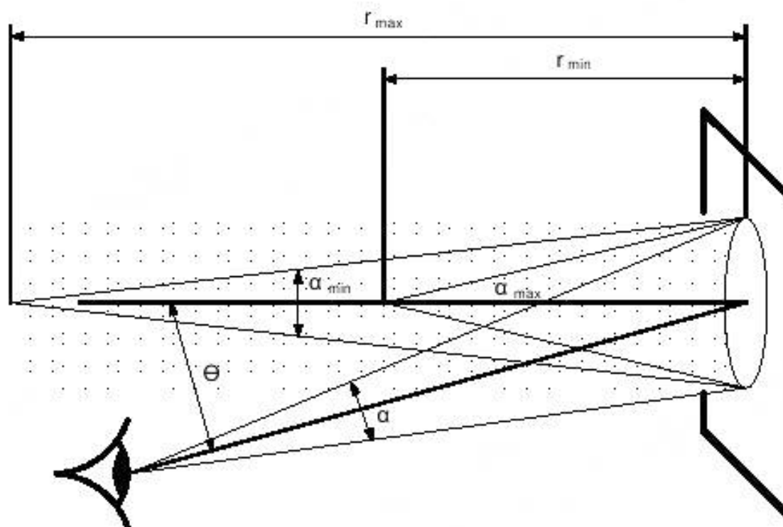
Рисунок 10 — Условия для просмотра распределенного источника
