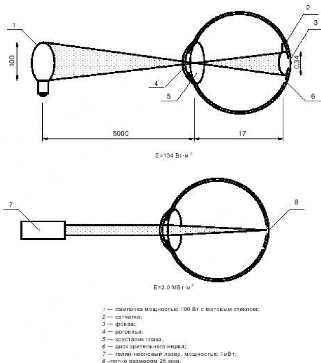
Рисунок 2 — Поперечное сечение глаза, показывающее сравнение плотности облучения сетчатки для изображения лампы мощностью 100 Вт и идеальной дифракции, ограничено пятно от гелий-неонового лазера энергией 1 мВт
