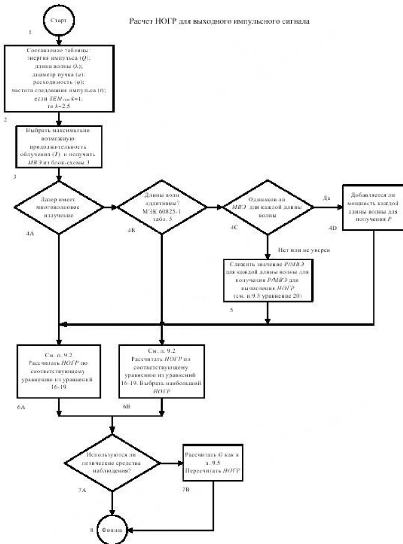
Блок-схема 2. Расчет НОГР для выходного импульсного сигнала
