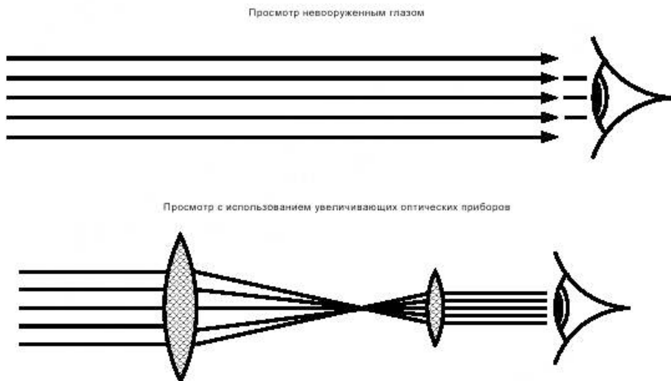
Рисунок 7 — Эффект от просмотра коллимированного пучка с использованием увеличительной оптики
