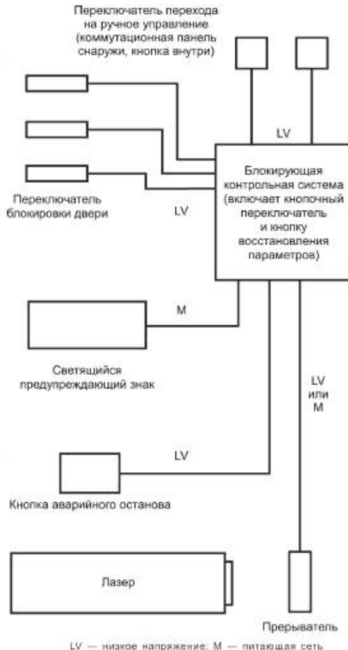
Рисунок A.2 — Система блокировки без запираания
