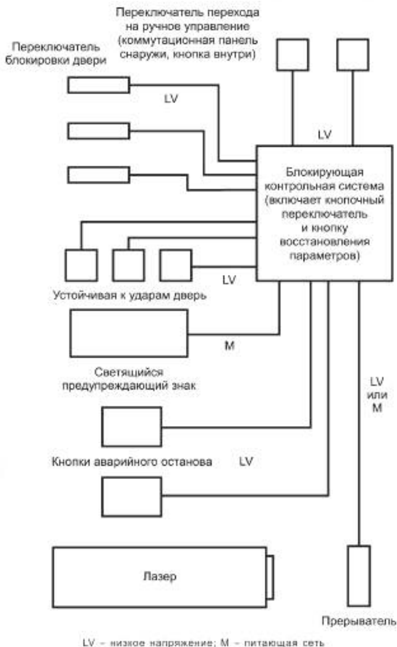
Рисунок A.3 — Система блокировки с запиранием
