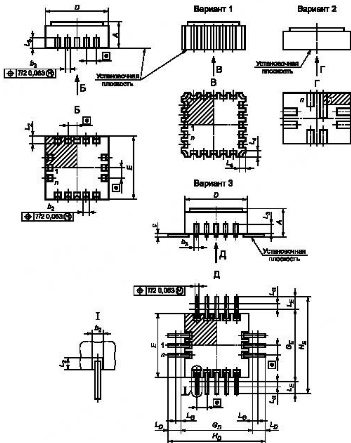
Рисунок 16 — Микросхемы в корпусах подтипа 51
