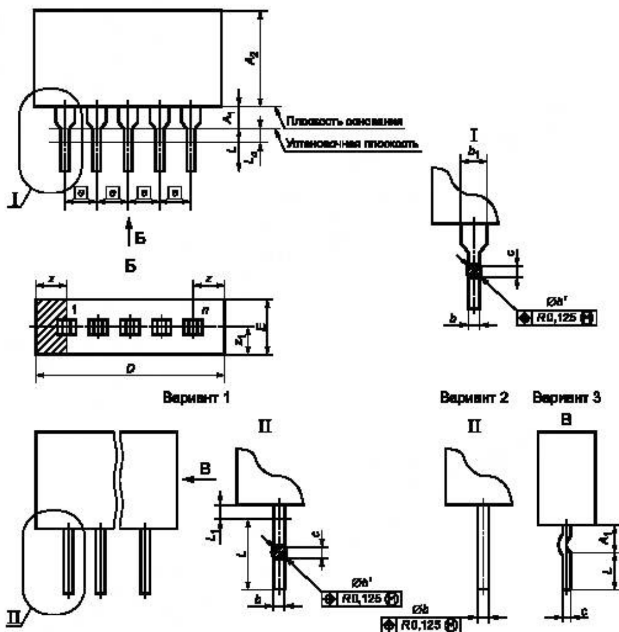
Рисунок 1 — Микросхемы в корпусах подтипа 11
