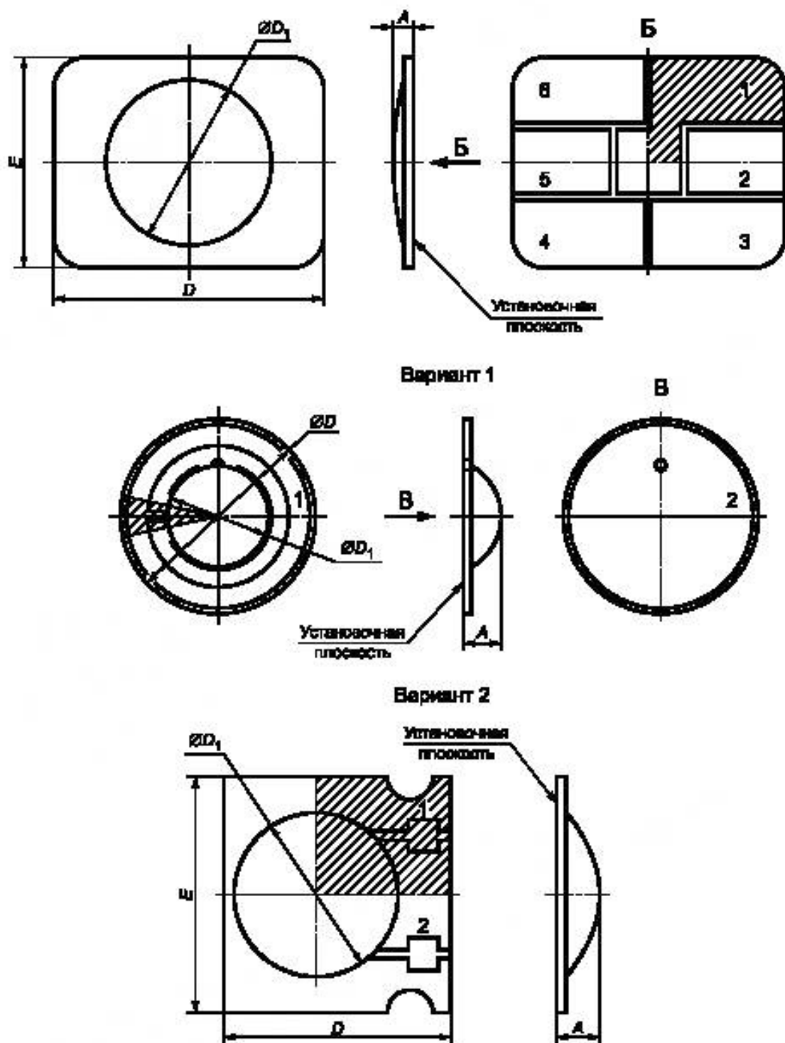
Рисунок 20 — Микросхемы в корпусах подтипа 71
