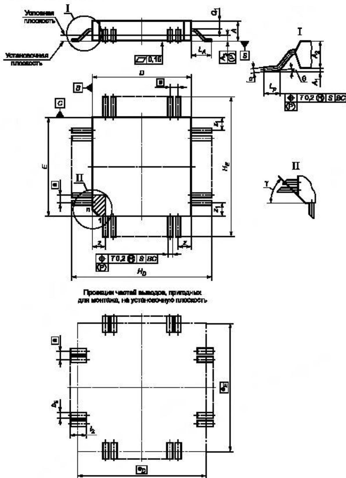
Рисунок 14 — Микросхемы в корпусах подтипа 44
