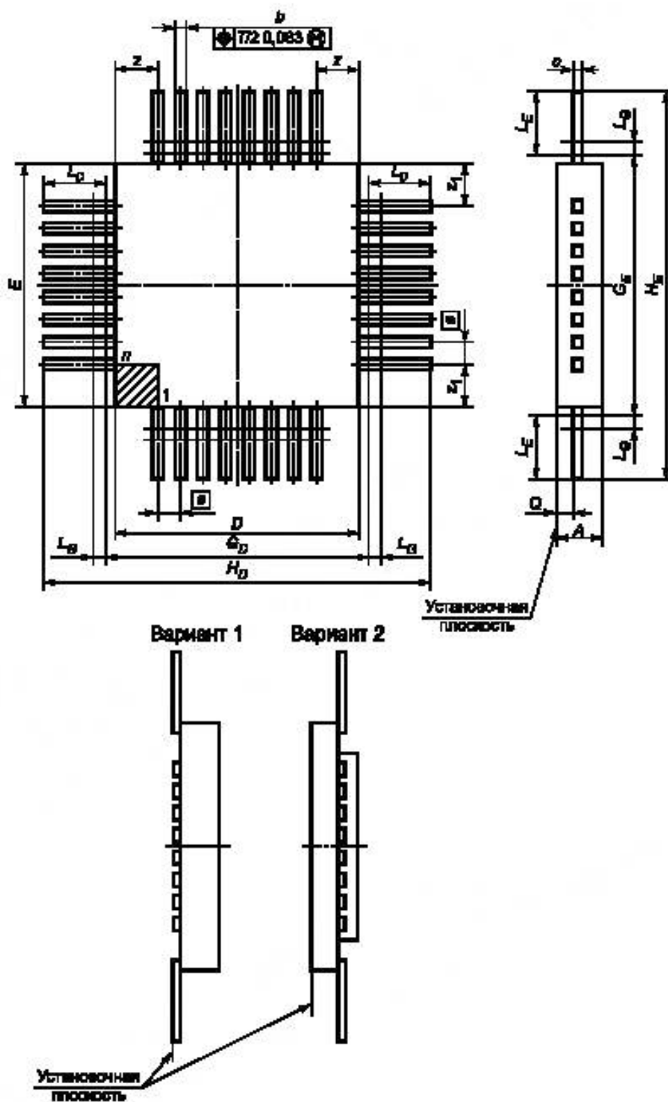
Рисунок 12 — Микросхемы в корпусах подтипа 42
