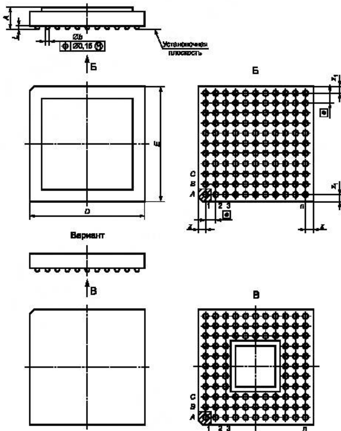
Рисунок 21 — Микросхемы в корпусах подтипа 81
