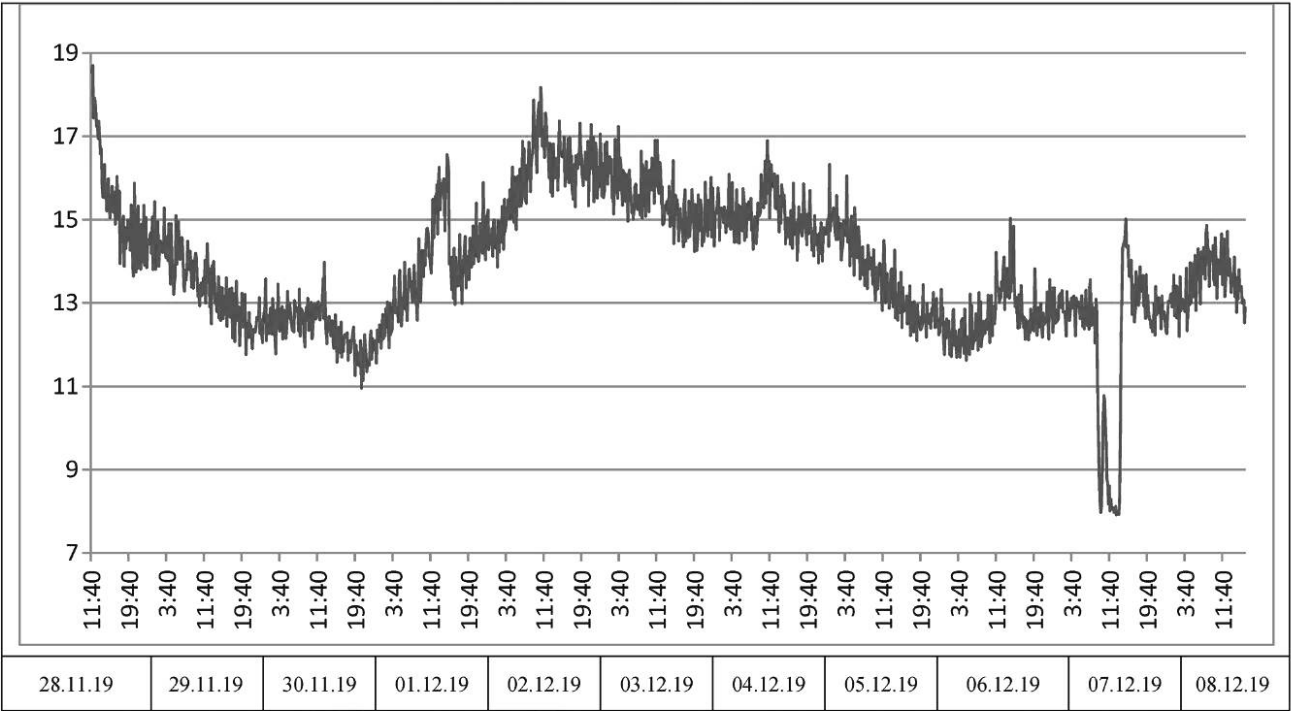
Рисунок 0.2.3 — График значений средней плотности теплового потока через стену, Вт/м²
