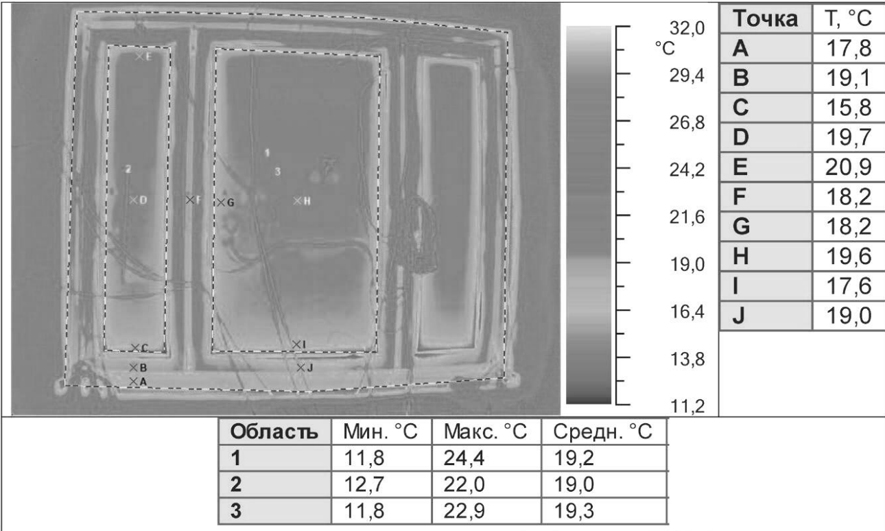
Рисунок 0.1.1 — Распределение температурных полей на испытываемой конструкции
