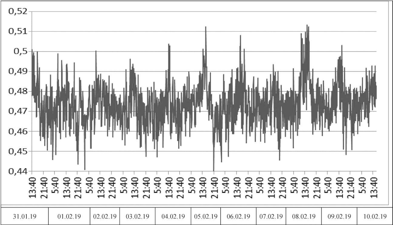
Рисунок 0.1.7 — График значений приведенного сопротивления теплопередаче стеклопакета, \text{м}^2 \cdot ^\circ\text{C}/\text{Вт}
