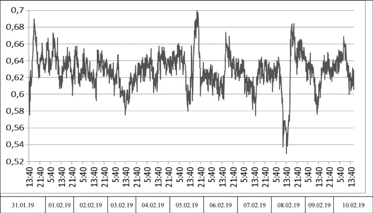
Рисунок 0.1.5 — График значений приведенного сопротивления теплопередаче профиля коробки, м² · °C/Вт
