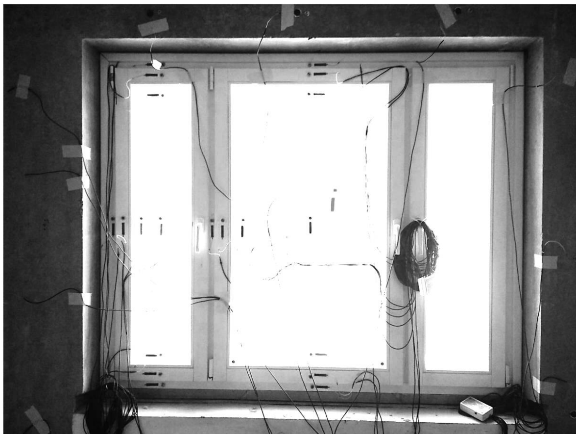
Фото 0.1. Оконный блок по оси 9 в осях Е—И на 3-м этаже 1-й секции с датчиками измерения плотности теплового потока и температуры.
