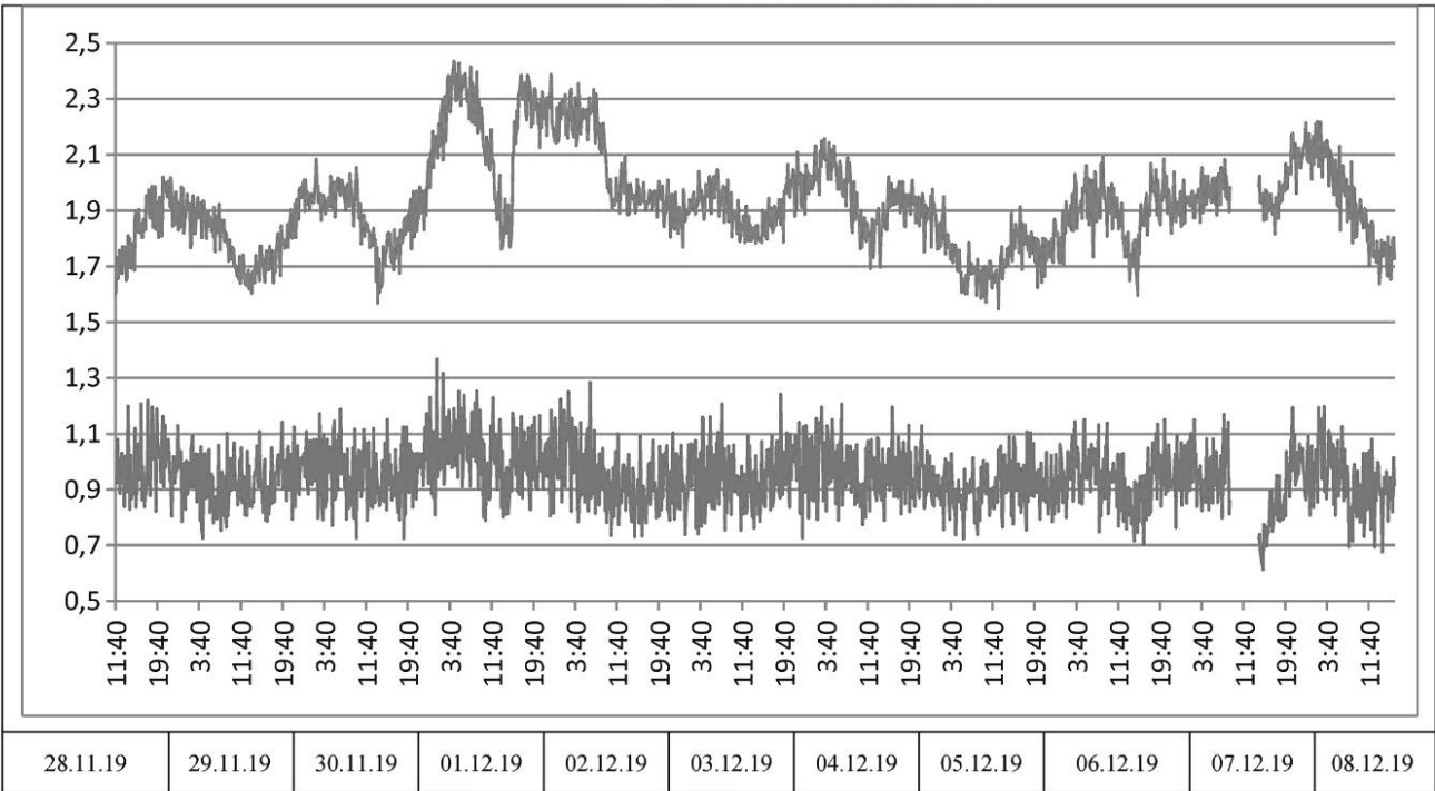
Рисунок 0.2.5 — График максимальных и минимальных значений приведенного сопротивления теплопередаче стены, \text{м}^2 \cdot ^\circ\text{C}/\text{Вт} Максимальное значение приведенного сопротивления теплопередаче стены за период измерений составляет 1,93 \text{ м}^2 \cdot ^\circ\text{C}/\text{Вт} ; минимальное значение приведенного сопротивления теплопередаче стены за период измерений — 0,95 \text{ м}^2 \cdot ^\circ\text{C}/\text{Вт} .
