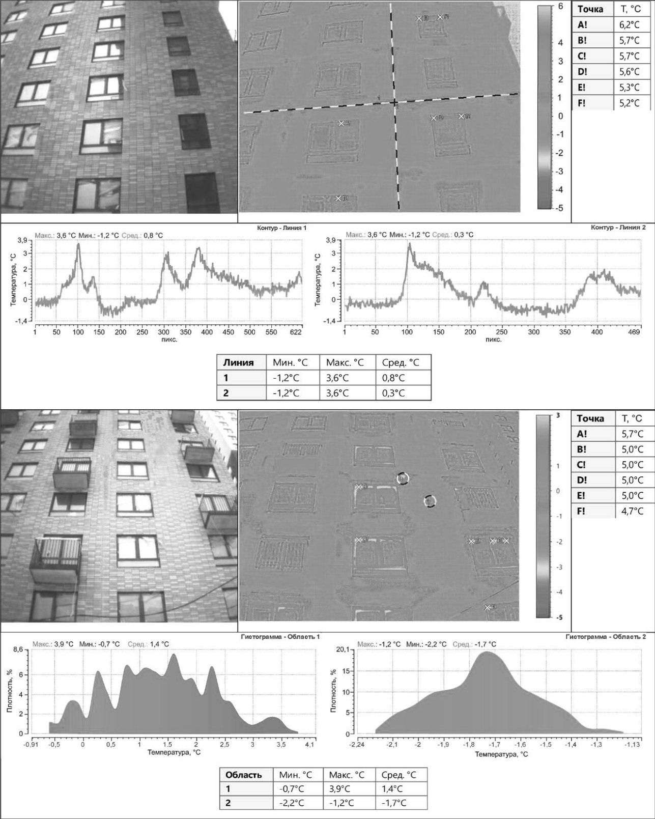
Рисунок 0.0.1 — Фасад здания в осях 1—4 по оси А
