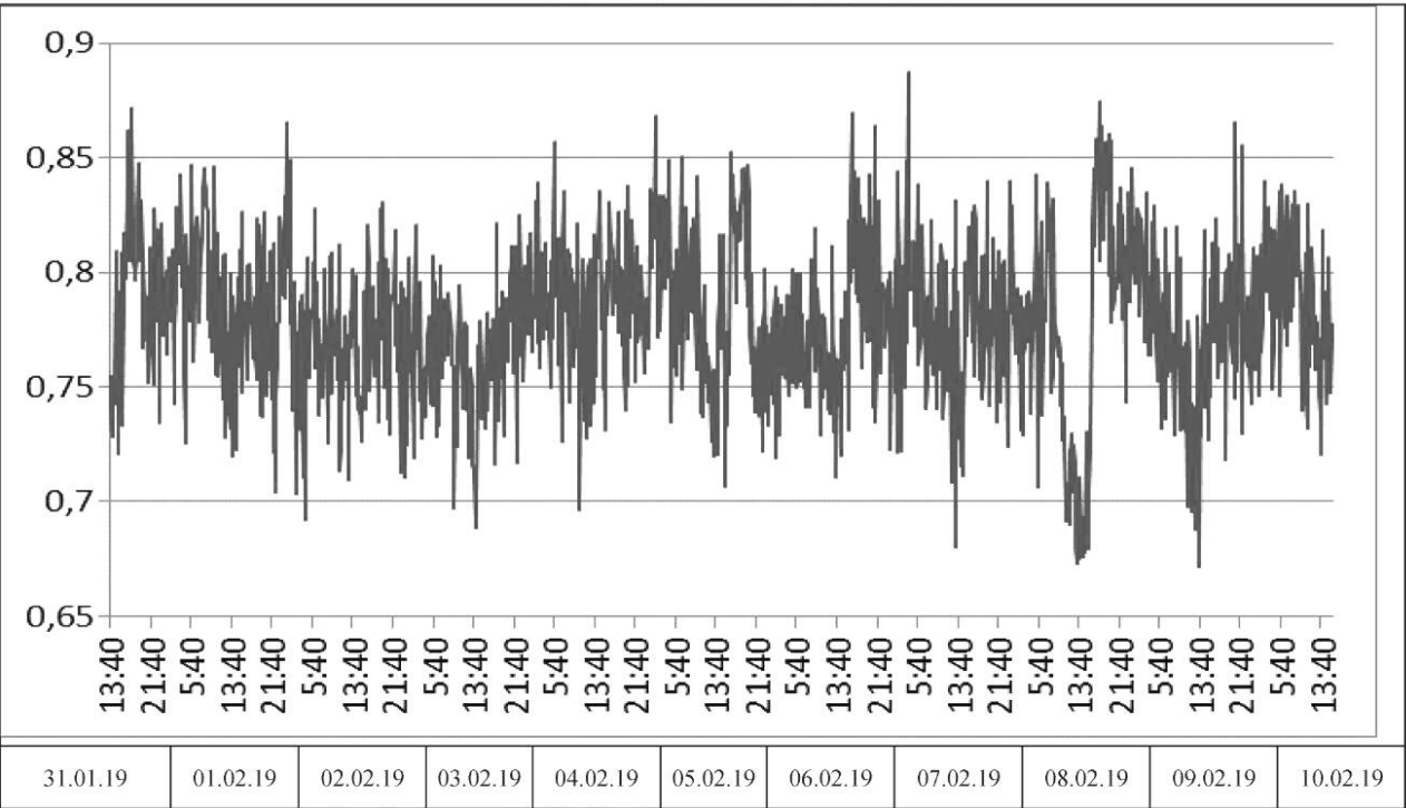
Рисунок 0.1.6 — График значений приведенного сопротивления теплопередаче профиля створок, м² · °C/Вт
