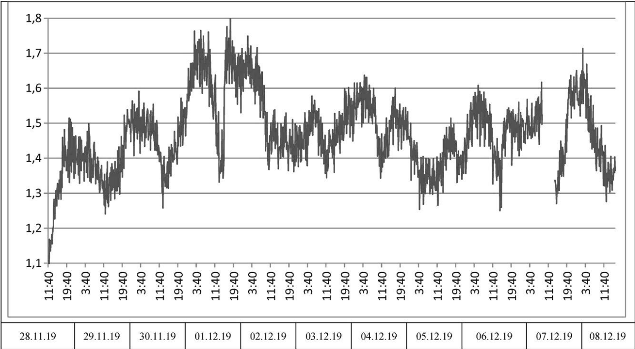
Рисунок 0.2.4 — График значений приведенного сопротивления теплопередаче фрагмента стены, \text{м}^2 \cdot ^\circ\text{C}/\text{Вт} Среднее значение приведенного сопротивления теплопередаче с учетом доверительной вероятности 99,7 % за период измерений составляет (1,47 \pm 0,11) \text{ м}^2 \cdot ^\circ\text{C}/\text{Вт} .
