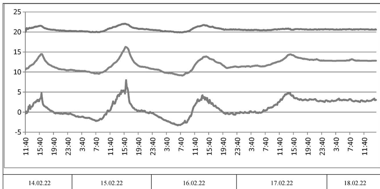
Рисунок А.9 — Графики значений температур внутреннего воздуха (верхняя линия), наружного воздуха (нижняя линия) и поверхности в точке а на стеклопакете, °С
