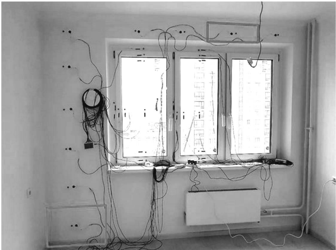
Фото 0.2. Стена (тип 1) с датчиками измерения теплового потока и температуры в осях 1—2 по оси В на 7-м этаже. Красным контуром выделена наиболее теплопроводная зона, синим — наименее.
