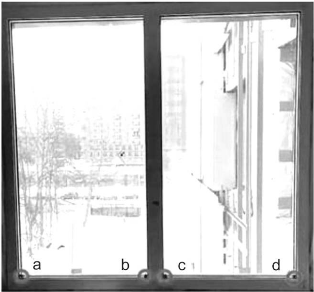
Фото оконного блока с установленным измерительным оборудованием
