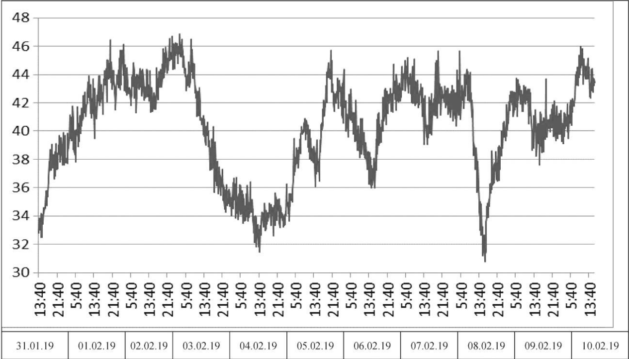
Рисунок 0.1.3 — График значений средней плотности теплового потока через испытываемую конструкцию оконного блока, Вт/м²
