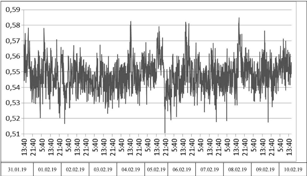
Рисунок 0.1.4 — График значений приведенного сопротивления теплопередаче оконного блока, м² · °C/Вт
