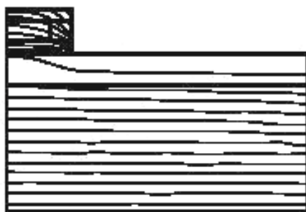
Рисунок 4 — Изотермы ( \delta\theta = 0,05 °C) для установленного на стене тепломера, обшитого и защищенного (цилиндрическое сечение)
