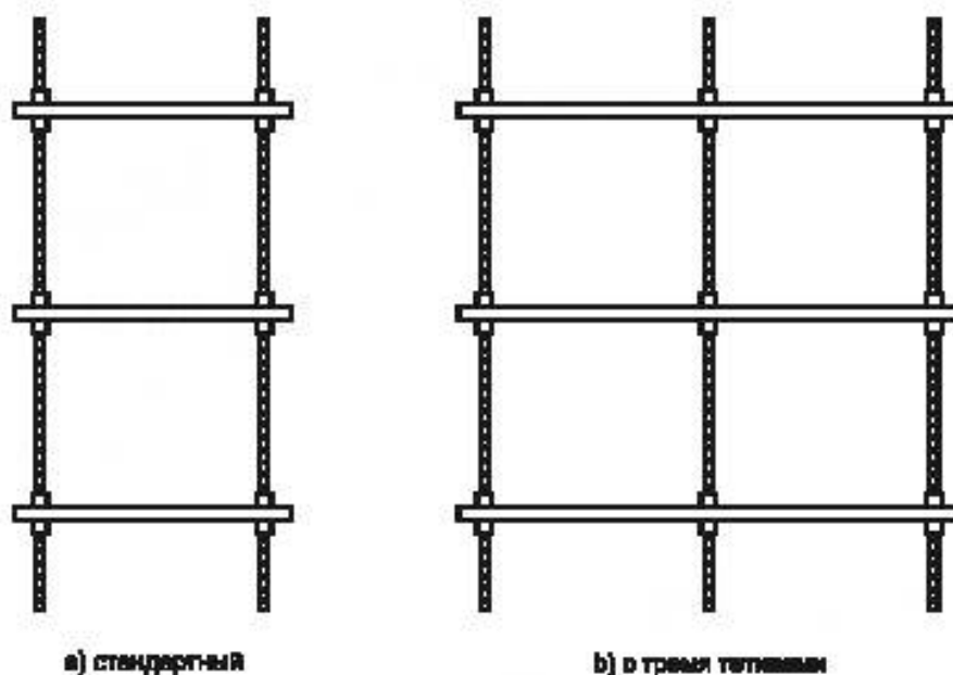
Рисунок 1 — Штурмтрапы
