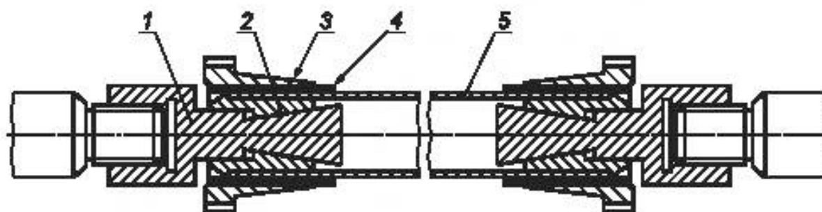
1 — шпилька; 2 — раздвигающаяся часть захвата; 3 — втулка; 4 — фиксирующий пояс; 5 — образец
