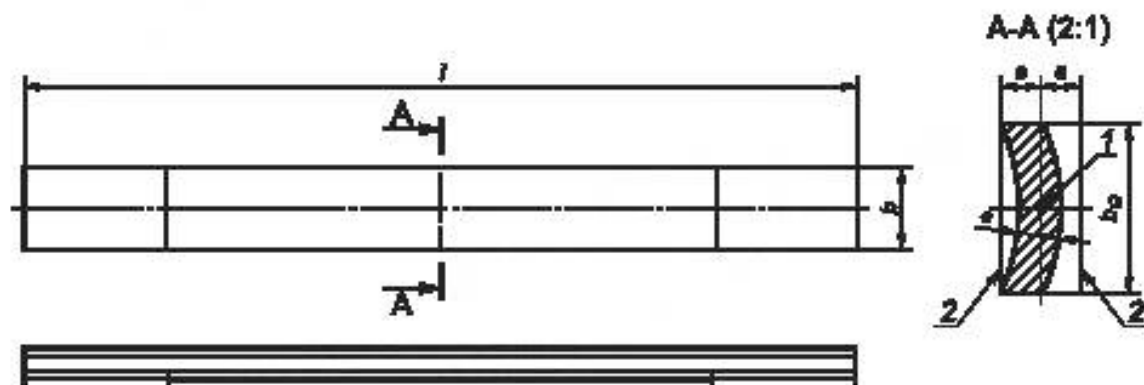
Рисунок 2 — Образец в форме лопатки (для метода А)
