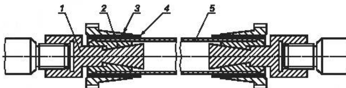
1 — шпилька; 2 — сегментированные захваты; 3 — ступка; 4 — укрепляющий пояс; 5 — образец для испытания
