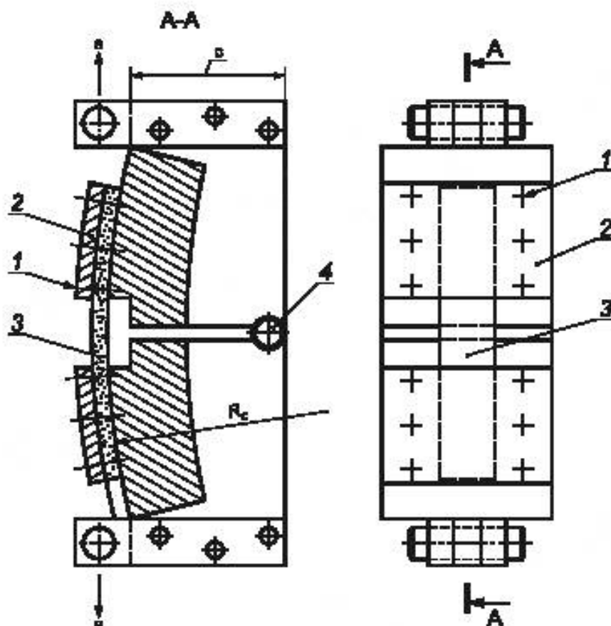
1 — место крепления образца болтом; 2 — прижимная пластина; 3 — образец; 4 — шарнир; R_c — радиус кривизны опорных пластин; s — регулируемое расстояние
