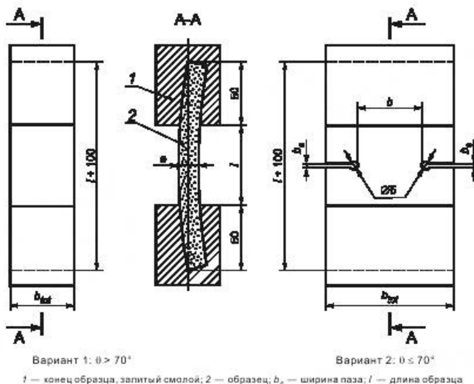
Рисунок 5 — Образцы для испытания (метод В)
