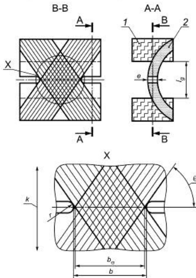
Рисунок 9 — Схема крепления образца (метод Е)
