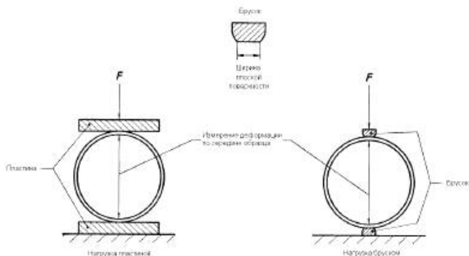
Рисунок 2 – Схема установки испытываемого образца в опорных площадках
